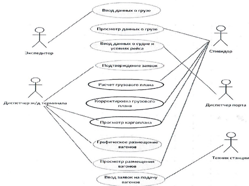
Рис.1 Діаграма прецедентів
