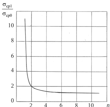
Рис. 2. Зависимость отношения среднего напряжения, действующего в середине концентратора напряжений, к напряжению на бесконечном удалении от него к относительному значению радиуса сопряжения прерывистой конструкции или радиуса окружности выреза
