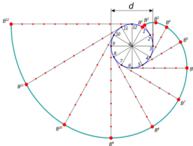
Рис. 12. Евольвента кола
