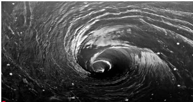
Рис.6. Спіралеподібні природні явища: а – вір на воді; б – повітряні маси циклона.
