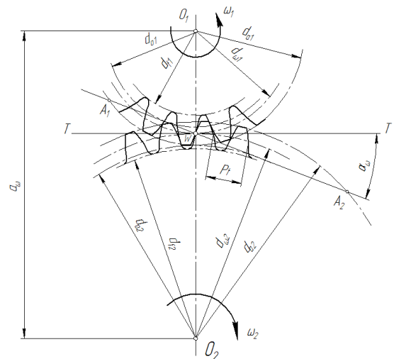
Рис. 13. Евольвентне зачеплення
