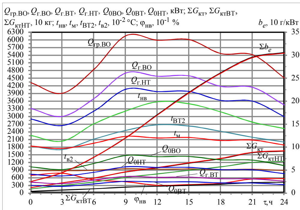
Рис. 3. Текущие значения температуры t_{нв} и относительной влажности \phi_{нв} наружного воздуха, температуры воздуха t_{ВТ2} на выходе из ВО ВТ и t_{В2} из ВО НТ , тепловых нагрузок Q_{0ВТ} на ВО ВТ , Q_{0НТ} на ВО НТ и Q_0 на весь ВО, соответствующего накопления конденсата за сутки \sum G_{ктВТ} , \sum G_{ктНТ} и \sum G_{кт} , тепловой нагрузки на градирни Q_{гр.ВО} системы оборотного охлаждения АБХМ и ЭХМ, суммарной по нарастающей за сутки удельной (приходящейся на 1 кВт мощности ГТУ) экономии топлива \sum b_e за счет охлаждения воздуха на входе ГТУ UGT 10000 (расход воздуха 40 кг/с) в течение суток (8.07.2015) для высокотемпературной ВО ВТ , низкотемпературной ВО НТ ступеней и всего двухступенчатого ВО: Q_{0ВТ} , Q_{0НТ} и Q_0 — для ВО ВТ , ВО НТ и всего ВО; \sum G_{ктВТ} , \sum G_{ктНТ} и \sum G_{кт} — для ВО ВТ , ВО НТ и всего ВО; проектные q_{0ВТ} = 10 \text{ кВт/(кг/с)} ; q_{0НТ} = 24 \text{ кВт/(кг/с)} ; q_0 = 34 \text{ кВт/(кг/с)}
