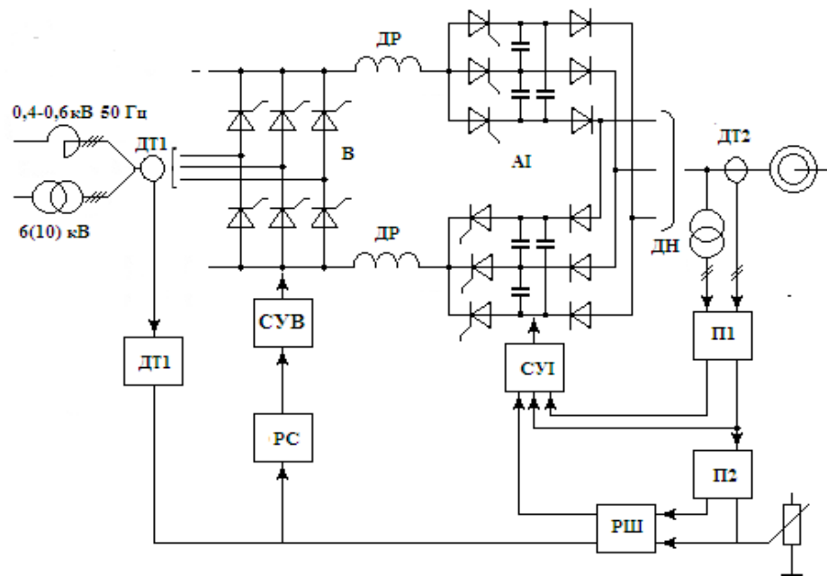
Рис. 4.5. Схема силової частини перетворювача частоти
