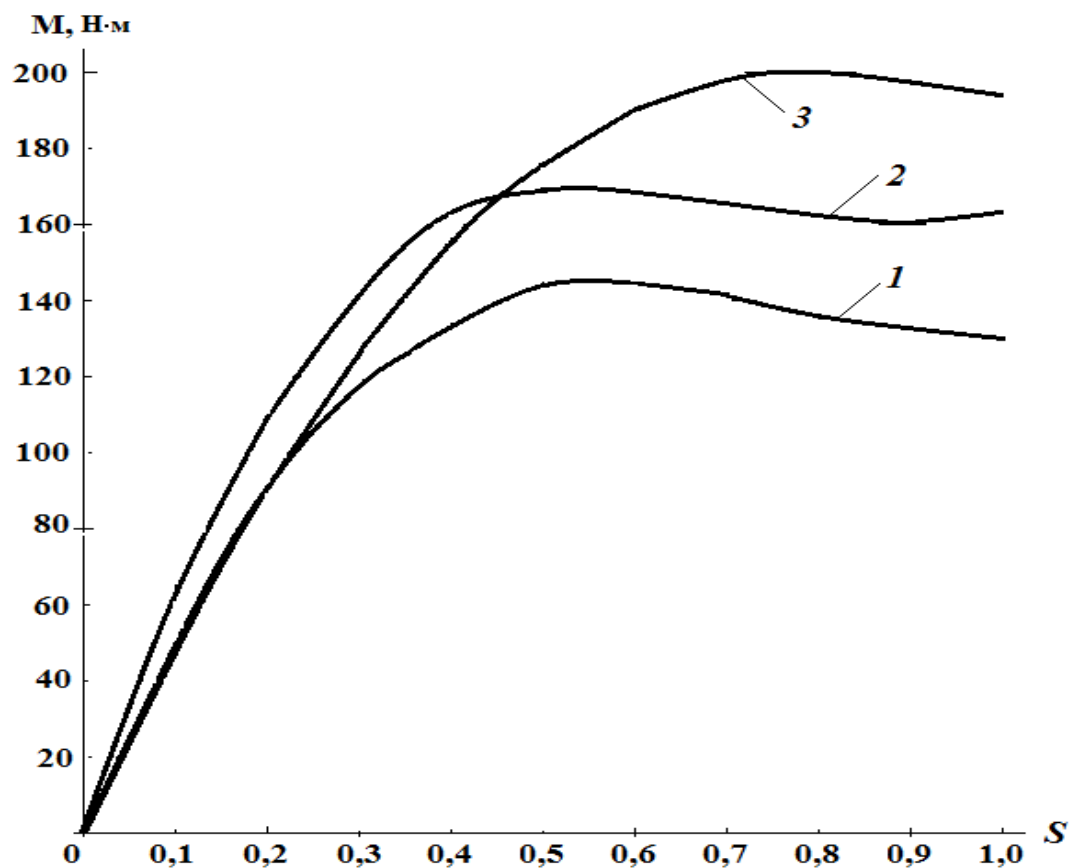
Рис. 4.7. Механічні характеристики (залежність моменту від ковзання)
