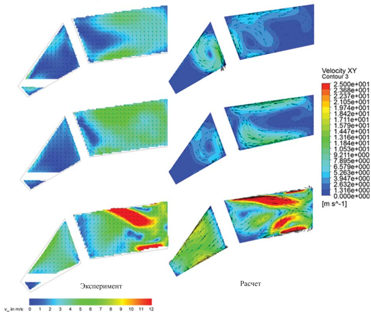
Рис. 4. Сравнение результатов и расчетов экспериментального исследования вторичных течений во вращающемся канале
