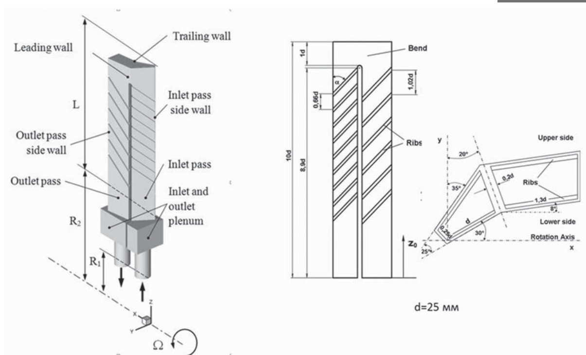
Рис. 3. Экспериментальный охлаждающий канал
