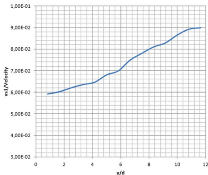
Рис. 6. Зависимость относительной тангенциальной скорости от относительной длины канала
