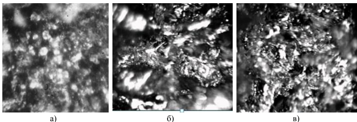
Рисунок 1 – Мікроструктура ( \times 350 ) електродугових покриттів на основі Св-АМг5, наповнених ( \approx 40\% об'ємн.):
