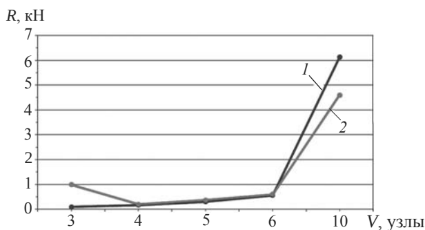
Рис. 11. Кривые буксировочного сопротивления: 1 — Модель 1; 2 — Модель 2
