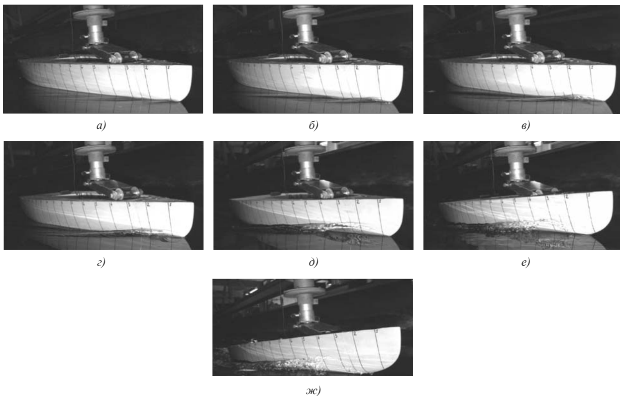
Рис. 13. Волнообразование Модели 2 при скорости хода:
