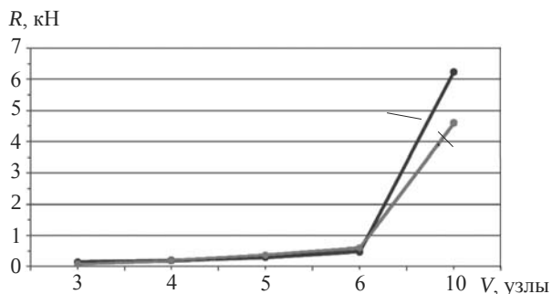
Рис. 6. Кривые буксировочного сопротивления:
