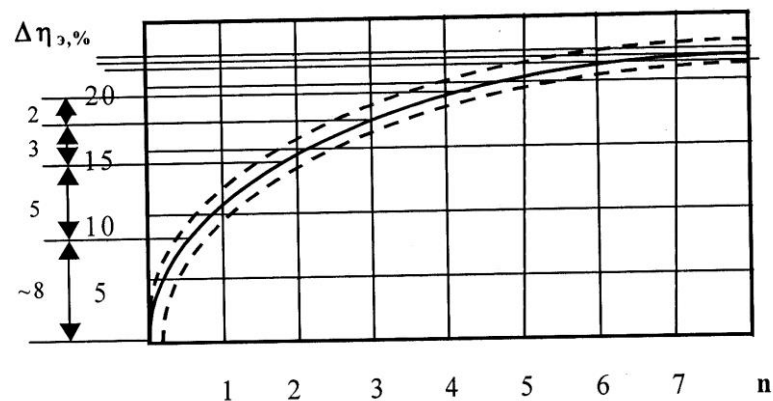
Рис. 7.5. Вплив кількості регенеративних підігрівачів на приріст ефективного ККД паротурбінної установки
