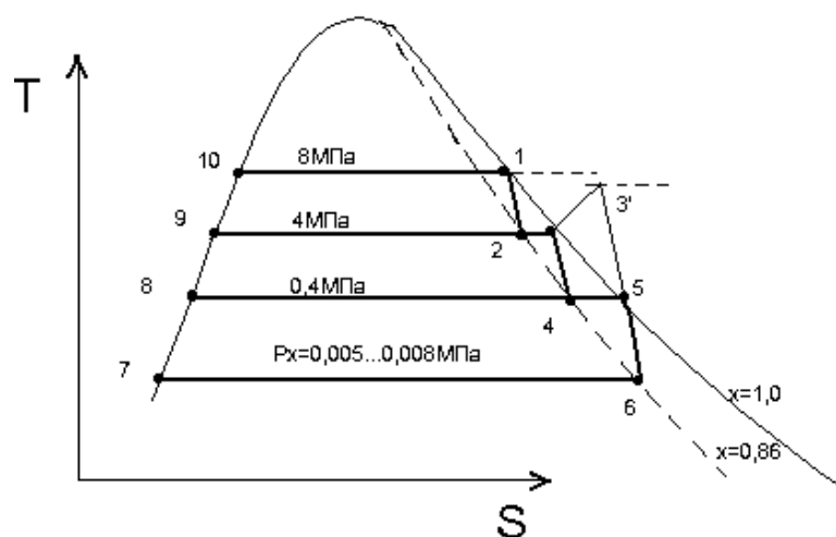
Рис. 6.5. Цикли паротурбінних установок на ядерному паливі
