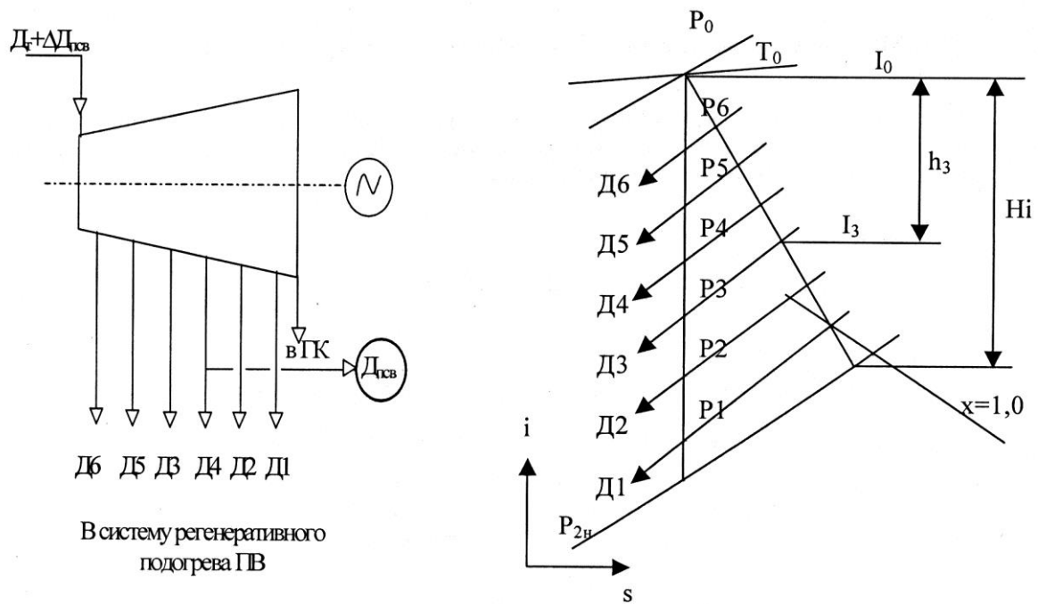
Рис. 9.3. До складання укрупненого матеріального балансу ТЕЦ
