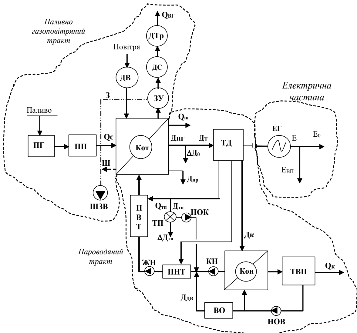
Рис. 3.2. Принципова технологічна схема електростанції
