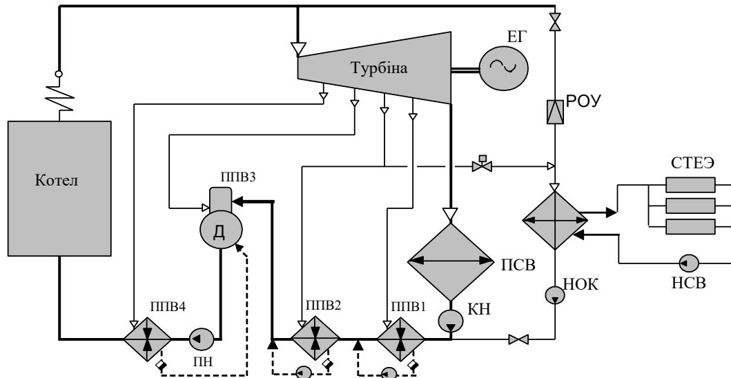
Рис. 4.7. Теплова схема ТЕЦ з регульованим відбором в турбіні
