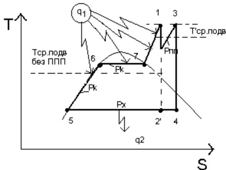
Рис. 6.1. Цикл ПТУ з проміжним перегрівом пари в s - T координатах
