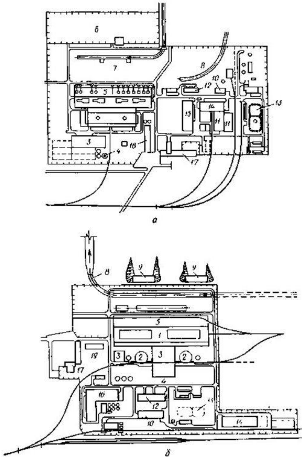
Рис. 11.5. Генплан АЕС із суміщеною (а – АЕС з ВВЕР 2×440 МВт) та розімкненою (б – АЕС з ВВЕР 2×1000 МВт) головною будовою
