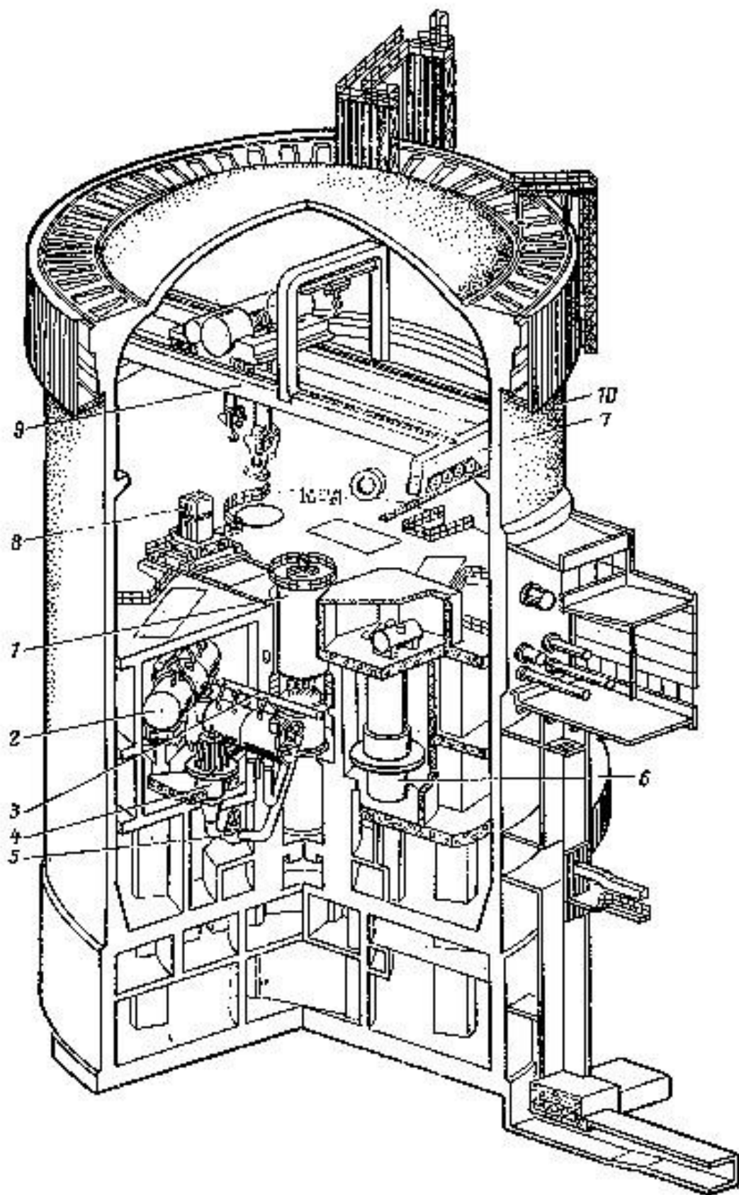
Рис. 12.8. Конструктивна схема реактора ВВЕР-1000
