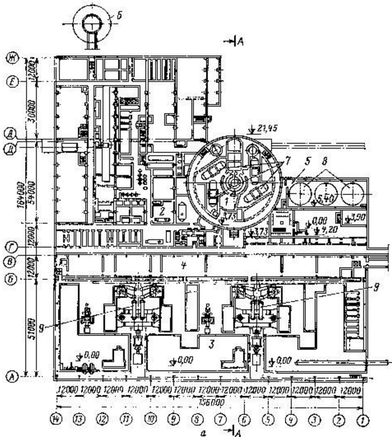
Рис. 12.7. Головна будівля АЕС: план (а) і розріз (б) – розімкнутого типу (АЕС з реактором ВВЕР-1000)
