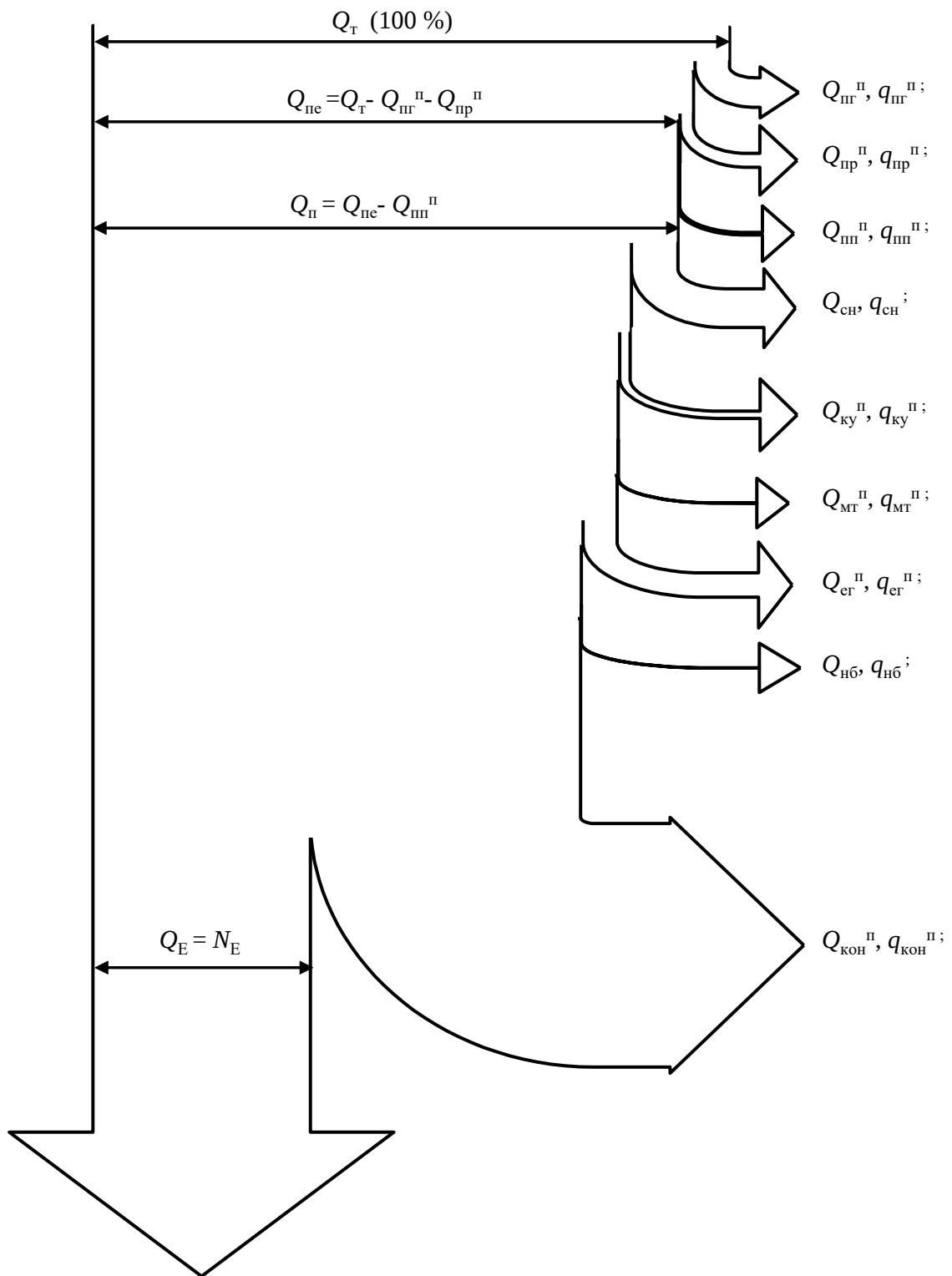
Рис. 9.4. Діаграма теплового балансу конденсаційної електростанції
