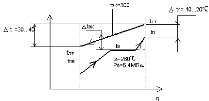
Рис. 6.4. Процеси теплообміну в парогенераторі двоконтурних ПТУ на ядерному паливі
