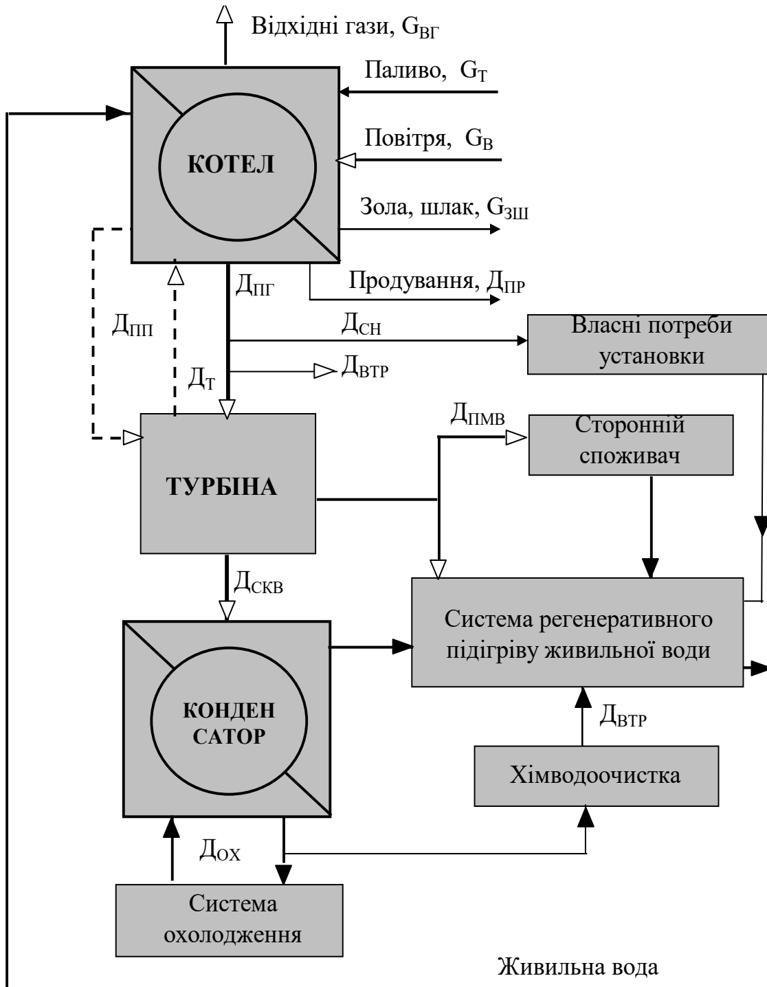
Рис. 9.1. Структурна схема розподілу матеріальних потоків (Коментарі до рисунка 9.1)
