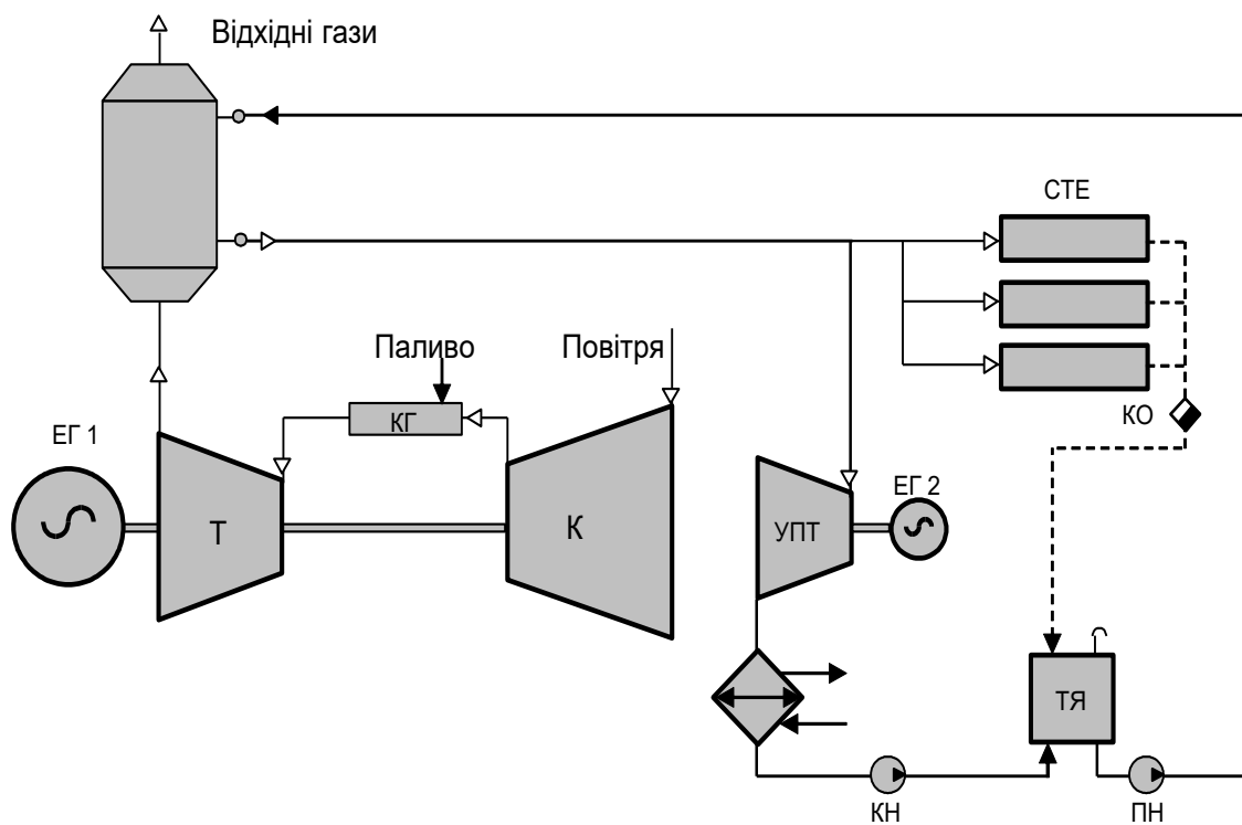
Рис. 4.10. Принципова теплова схема бінарної ГПТЕС
