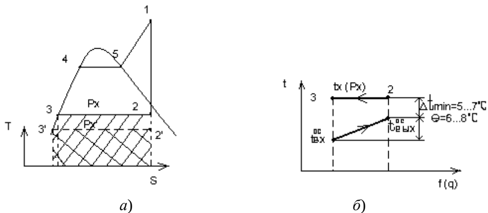
Рис. 5.4. До визначення впливу кінцевого тиску на теплову економічність установки
