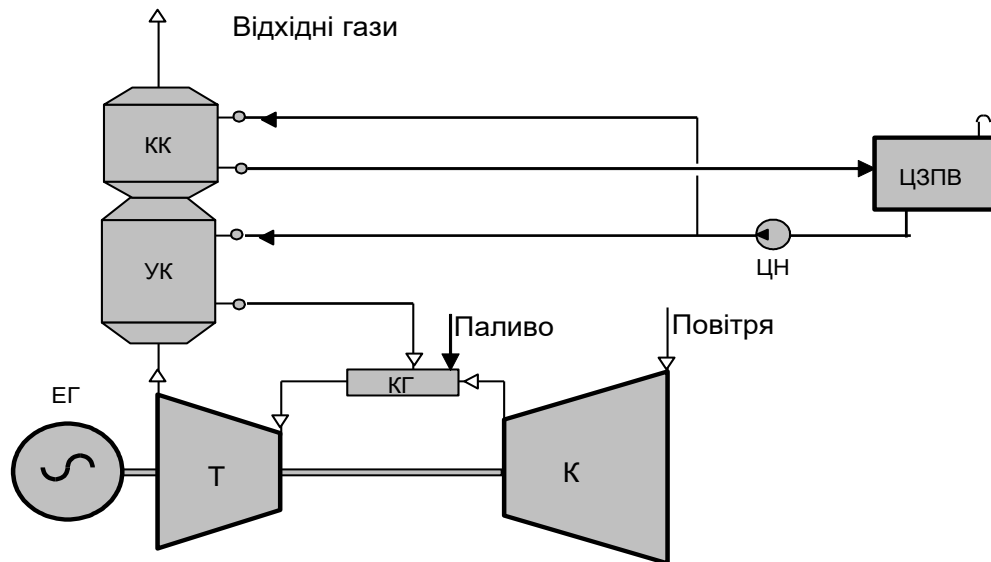
Рис.4.11. Принципова теплова схема контактної ГПТЕС
