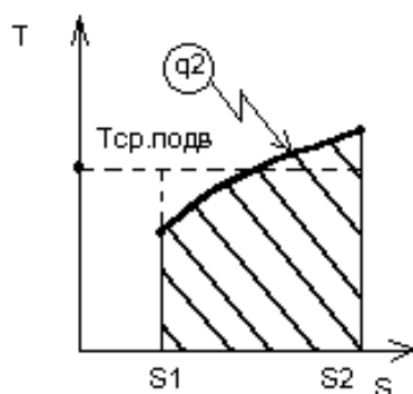
Рис. 5.2. До визначення середньотермодинамічної температури підведення теплоти
