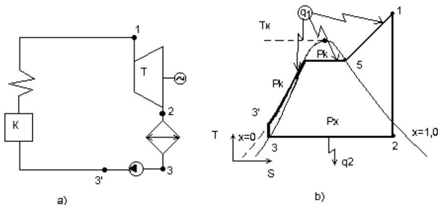
Рис. 5.1. Склад ідеалізованої паротурбінної установки і цикл, що лежить в основі її роботи
