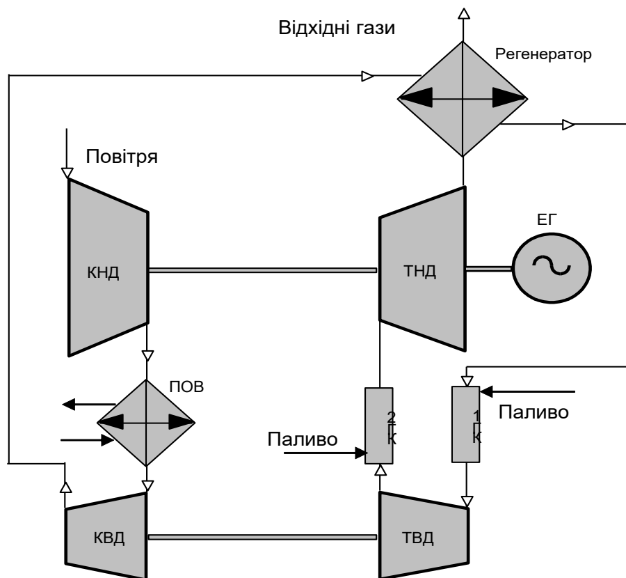
Рис. 4.9. Принципова теплова схема ГТЕС з регенерацією, проміжним охолодженням повітря і проміжним підведенням теплоти на лінії розширення
