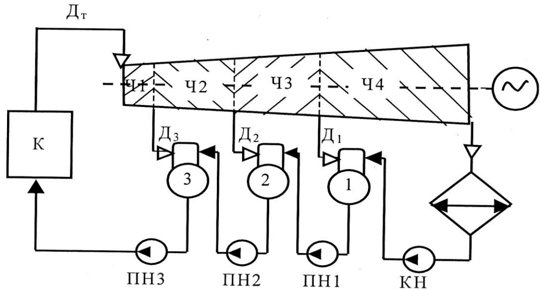
Рис. 7.4. Принципова теплова схема РТУ з підігрівниками живильної води змішувального типу
