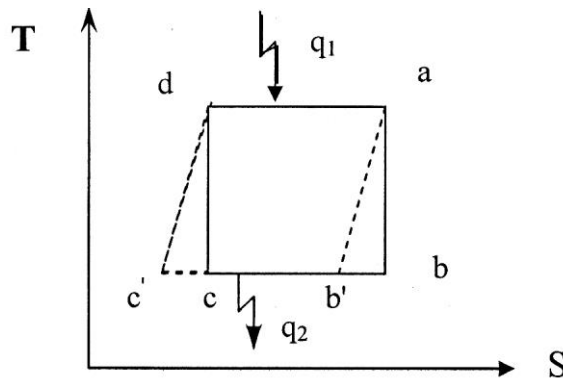
Рис. 7.1. Цикли Карно в s - T координатах
