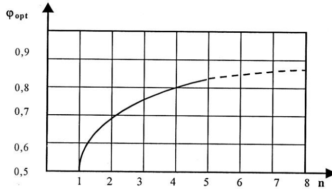
Рис. 7.7. Залежність оптимального ступеня регенерації теплоти в циклі від кількості регенеративних підігрівачів живильної води
