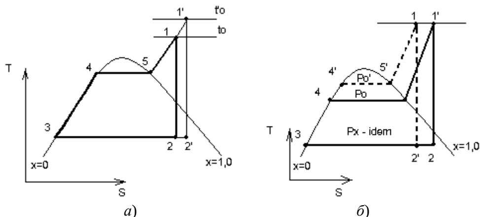
Рис. 5.3. До визначення впливу початкових параметрів температури пари на теплову економічність установки
