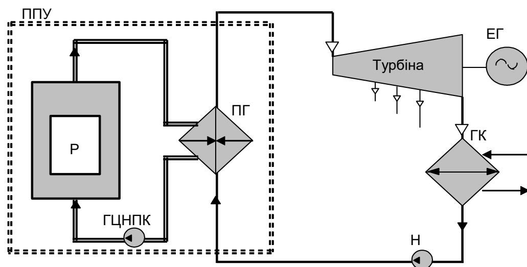
Рис. 4.4. Двоконтурна АЕС
