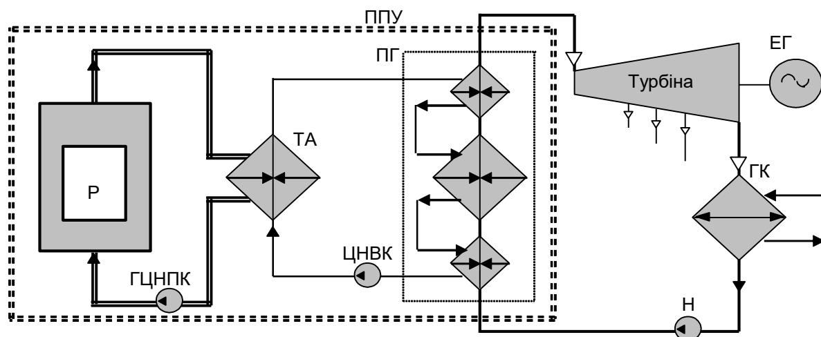
Рис. 4.5. Триконтурна АЕС
