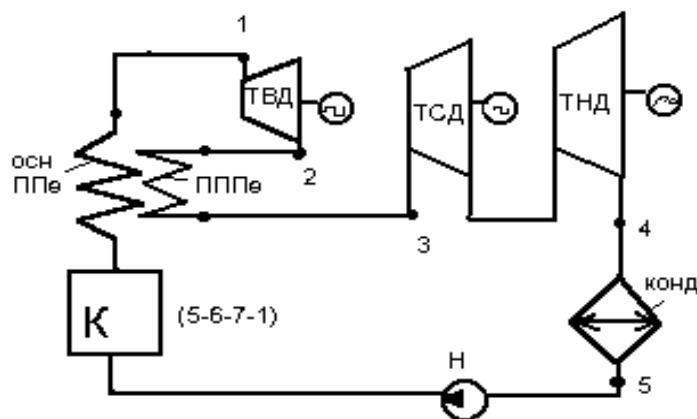
Рис. 6.2. Принципова теплова схемою РТУ з газовим проміжним перегрівом пари
