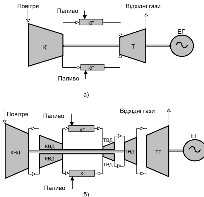
Рис. 4.8. Принципові схеми газотурбінних електростанцій а) одновальна ГТУ; б) тривальна ГТУ
