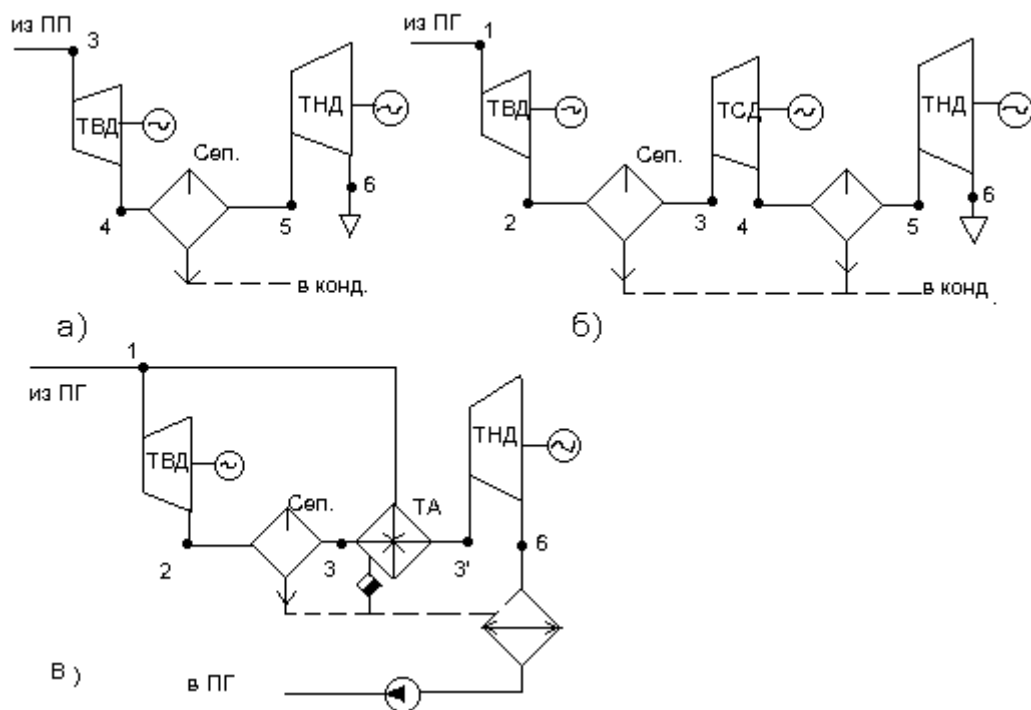
Рис. 6.6. Принципові схеми реалізації осушки пари в ПТУ проміжна сепарація пари – а) одноступенева; б) – двоступенева; проміжні сепарація і паровий перегрів пари – в)
