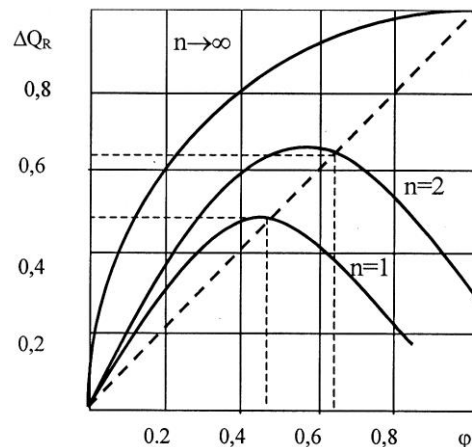
Рис. 7.6. Залежність відносної економії теплоти в циклі від ступеня регенерації
