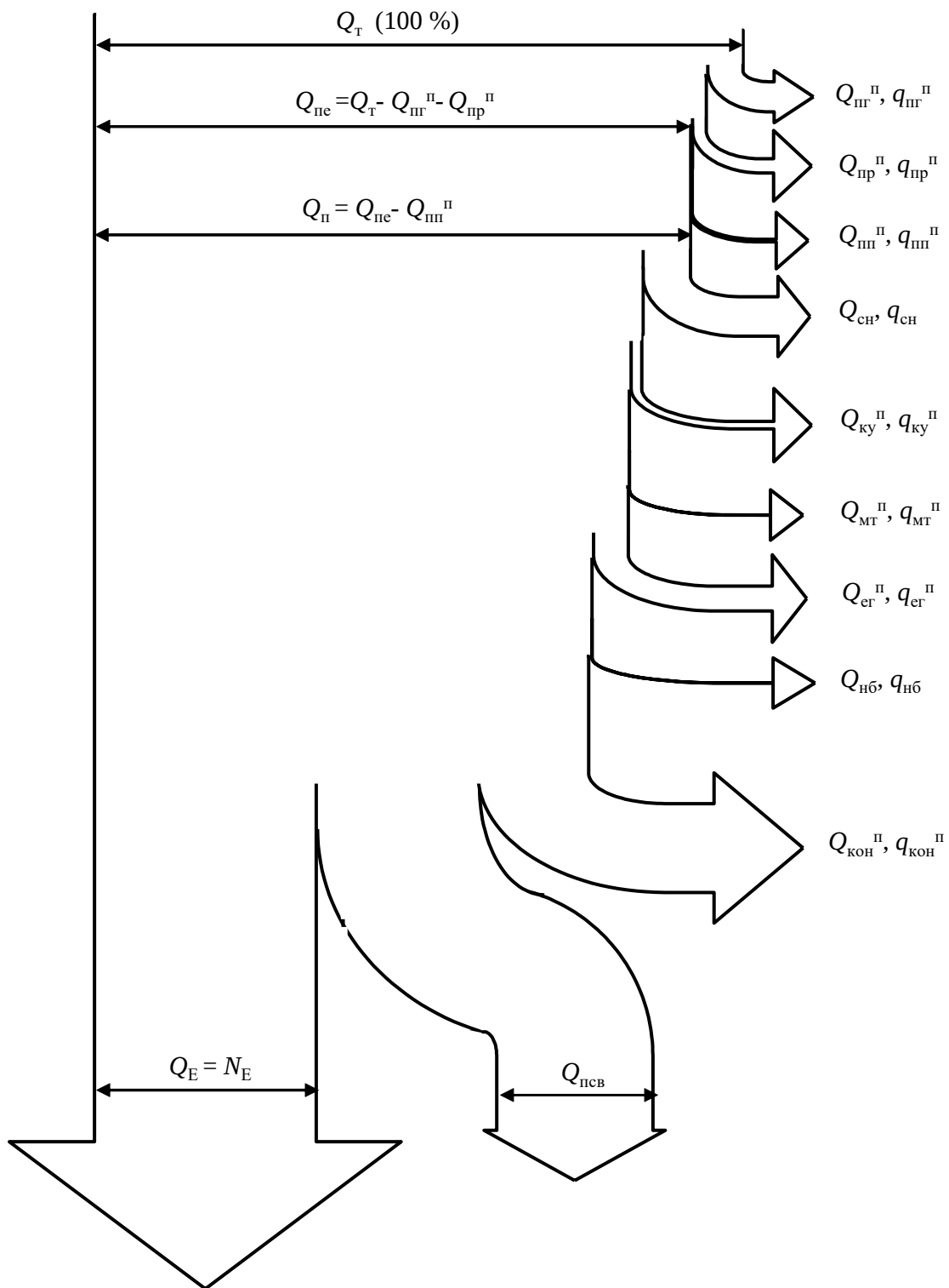
Рис. 9.5. Діаграма теплового балансу ПТУ, що прайює в складі ТЕЦ
