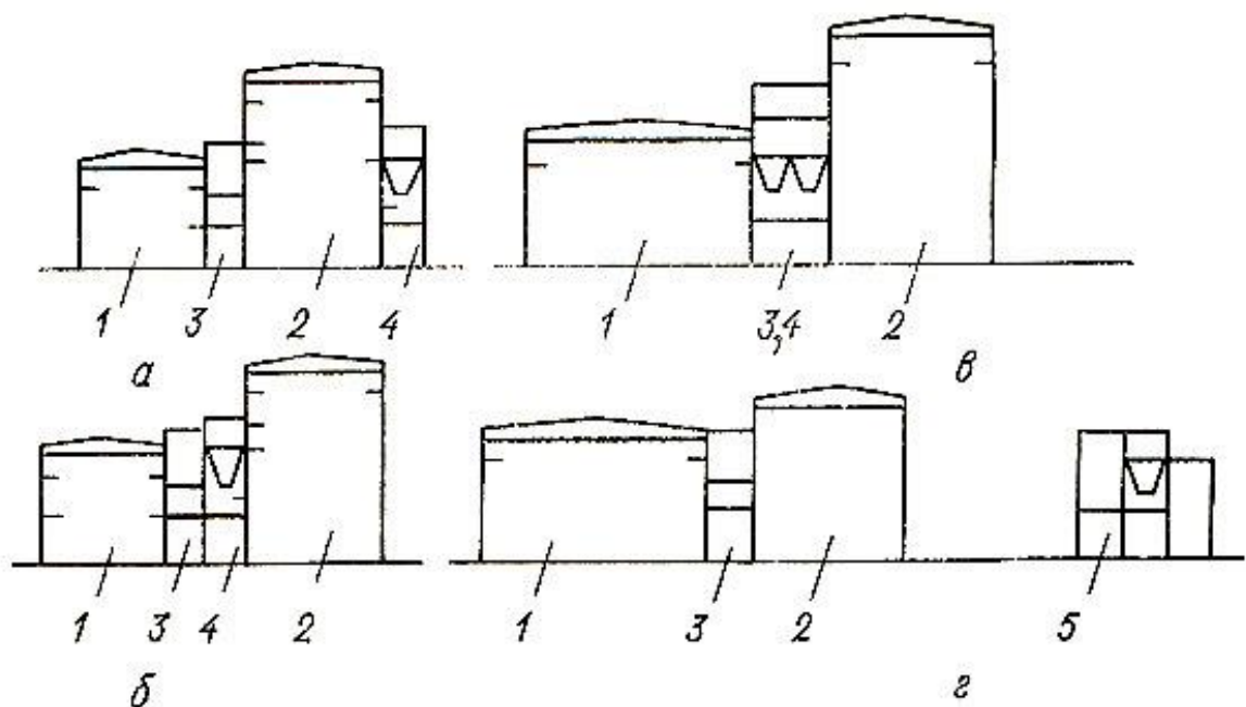
Рис. 12.1. Типи компоновок головної будови
