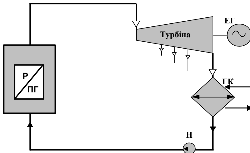
Рис. 4.3. Одноконтурна АЕС
