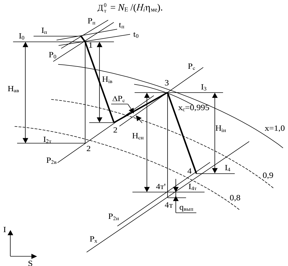
Рис. 8.3. Процес розширення пари в турбінному двигуні з проміжною сепарацією пари
