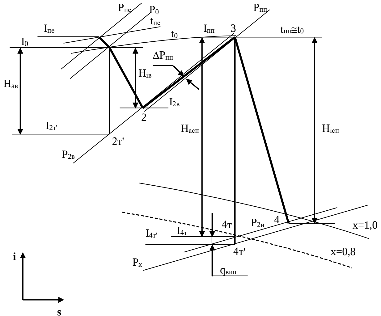
Рис. 8.2. Процеси розширення пара в турбінному двигуні (Коментар до побудови процесу розширення в турбіні аналогічний рис 8.1.)
