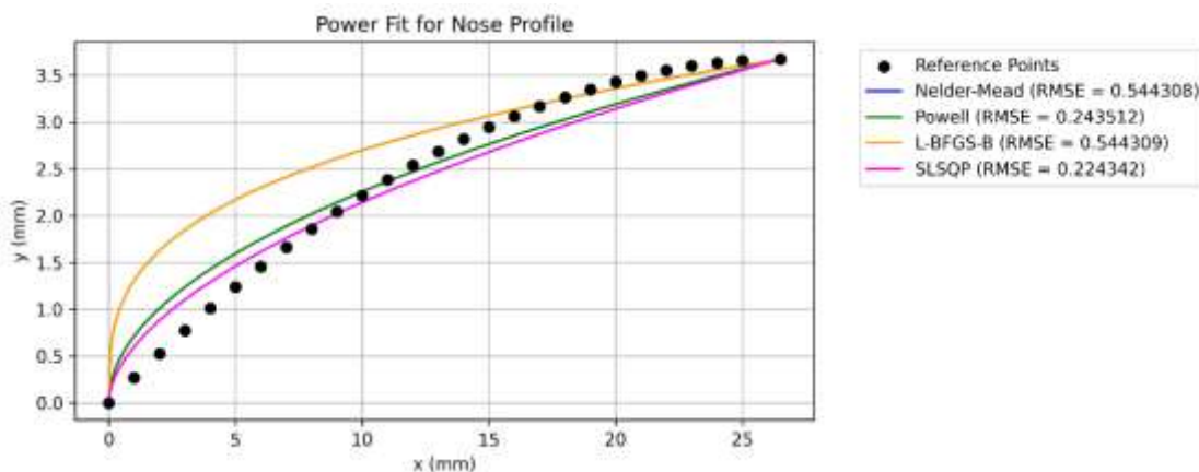
Рис. 4. Порівняння оптимізованих степеневих кривих для профілю носової частини снаряда
