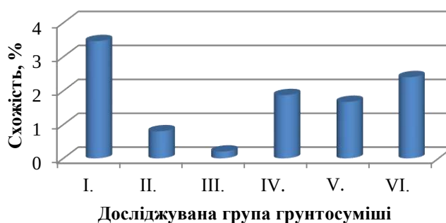
Рис. 1. Результати дослідження проростання насіння крес-салату на різних варіантах суміші ґрунту та червоного шламу
