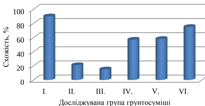
Рис. 2. Результати дослідження проростання зерен кукурудзи на різних варіантах суміші ґрунту та червоного шламу
