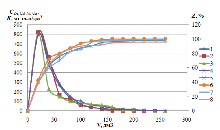
Рис. 8. Залежність вихідних концентрацій цинку (1), кадмію (2), нікелю (3) та міді (4), ступеня десорбції цинку (5), кадмію (6), нікелю (7) та міді (8) від об'єму пропущеного розчину 8 % сірчаної кислоти через катіоніт КУ-2-8 ( V_i = 20 \text{ см}^3 ) відповідно в \text{Zn}^{2+} (1; 5); \text{Cd}^{2+} (2; 6); \text{Ni} (3; 7); \text{Cu} (4; 8)
