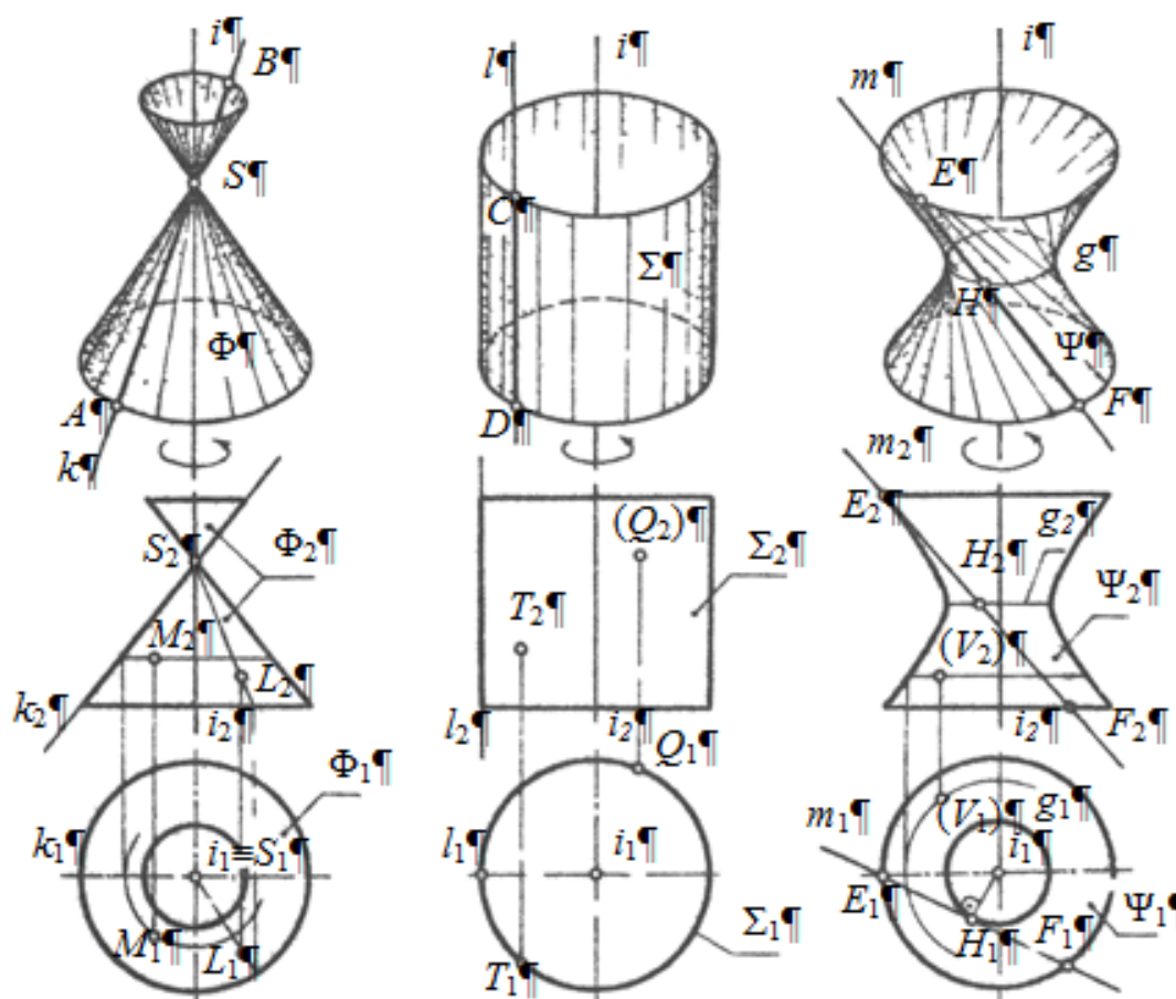
Рис. 1. Наочні зображення та проєкційні креслення конуса, циліндра та однопорожнинного гіперболоїда
