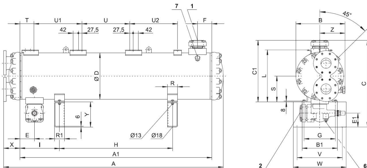
Рисунок 4.2. Габаритні розміри конденсатора фірми Bitzer серії K8503.B
