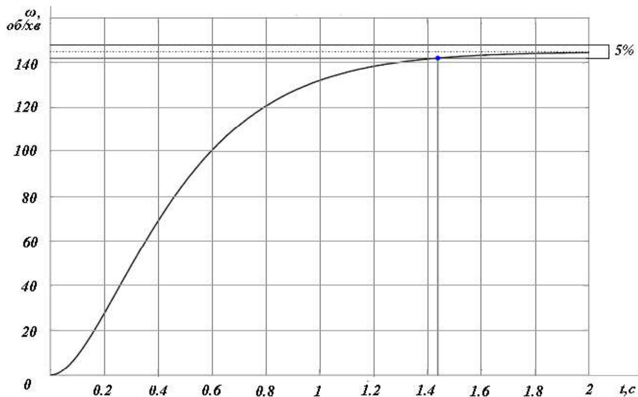
Рисунок 4.2 – Перехідний процес за кутовою швидкістю
