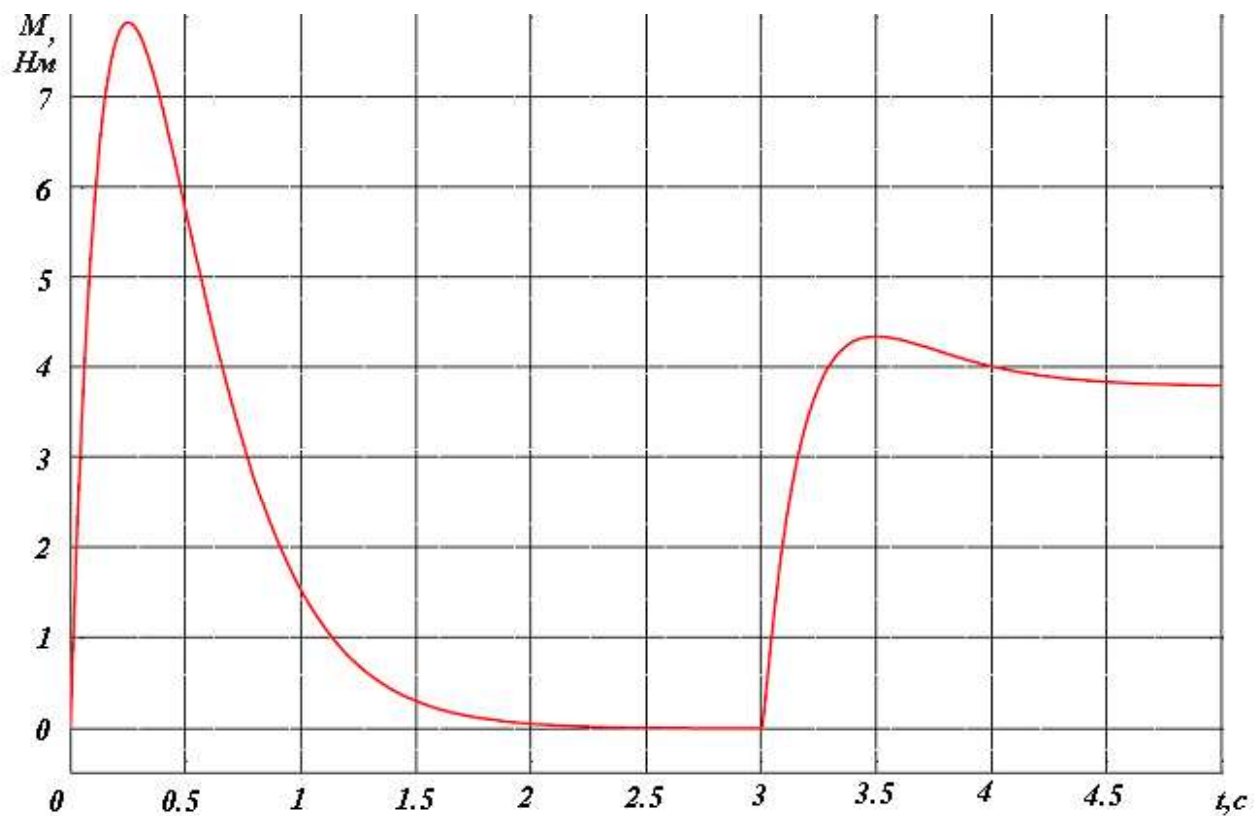
Рисунок 4.8 – Перехідний процес моменту на валу двигуна при стрибкоподібній зміні моменту 100% M_{ном}
