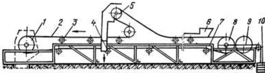
Рисунок 1.1 – Стрічковий конвеєр:
