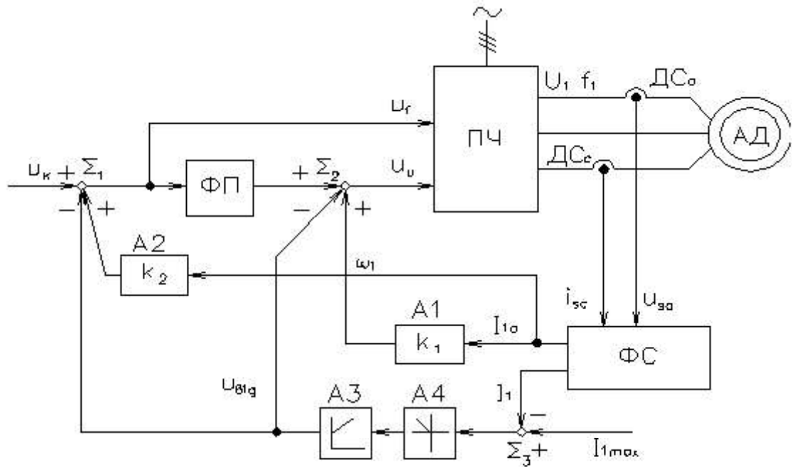
Рисунок 3.3 – Функціональна схема системи ПЧ-АД із зворотним зв'язком по струму статора
