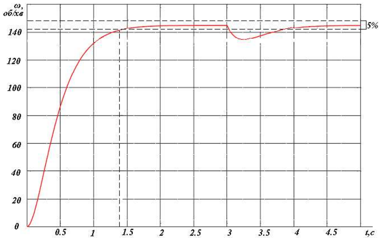
Рисунок 4.7 – Перехідний процес частоти обертання валу при стрибкоподібній зміні навантаження 100\% M_{\text{ном}}
