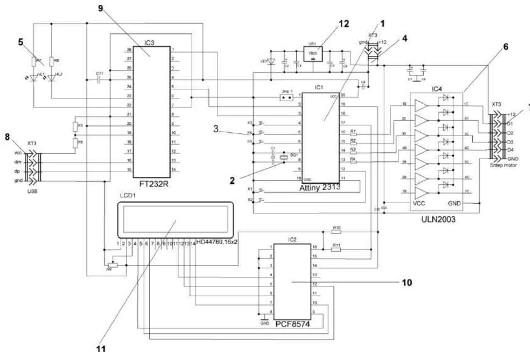
Рисунок 1 – принципова схема системи керування кроковими двигунами
