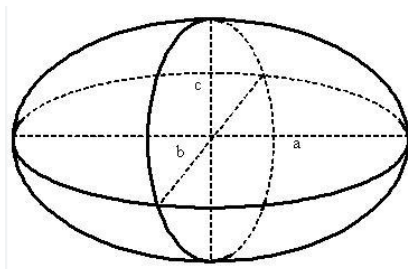
Рис.8. Зображення еліпсоїда
