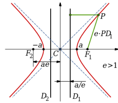
Рис. 6. Побудована гіпербола
