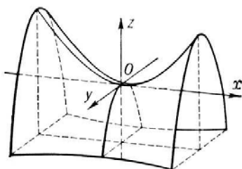
Рис.13. Гіперболічний параболоїд
