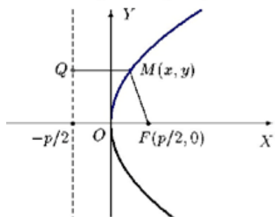
Рис. 4. Зображення параболі
