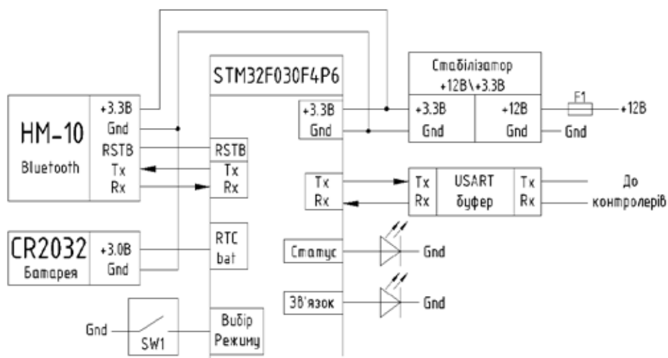
Рис. 2. Функціональна схема головного контролера
