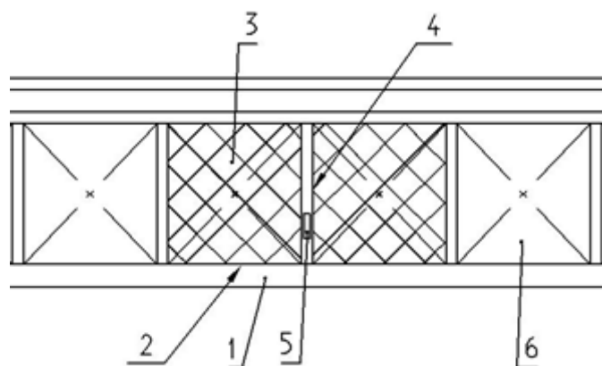
Рисунок 1 – Фрагмент вантажної зони: 1 – подвійне дно; 2 – вантажні танки, модернізовані під розігріті вантажі; 3 – теплова ізоляція; 4 – подвійна переборка; 5 – нагрівальне обладнання; 6 – танки для інших вантажів
