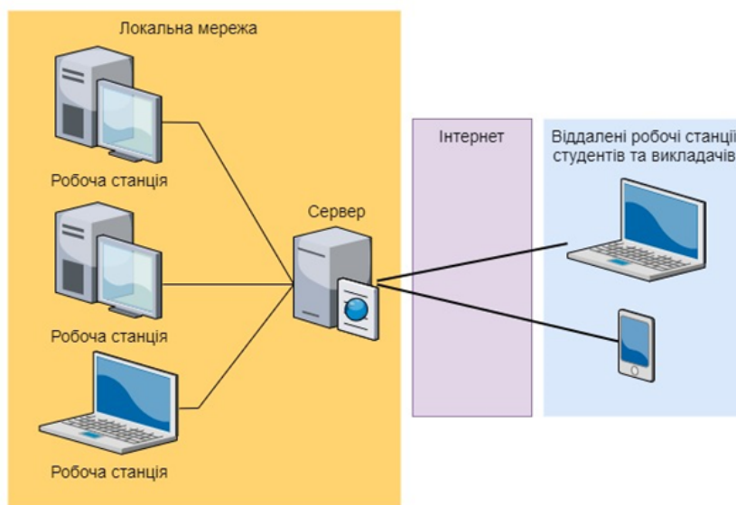
Рис. 2. Структурна схема практичного модуля системи
