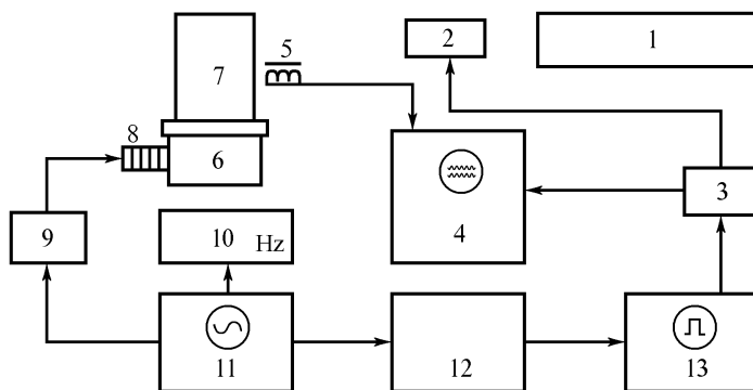
Рис. 1 – Функциональная схема вибростенда:
