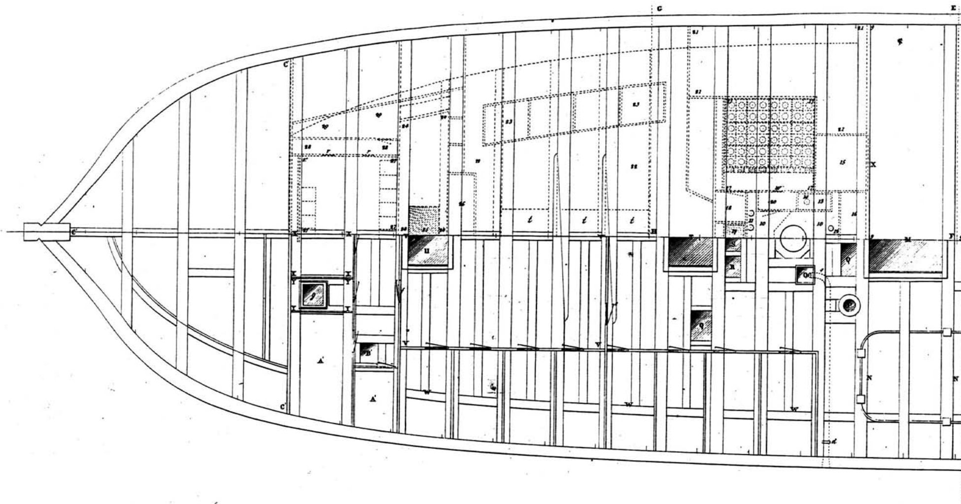
Разрез по линии S-H.
