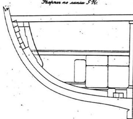
Разрез по линии S-H.
