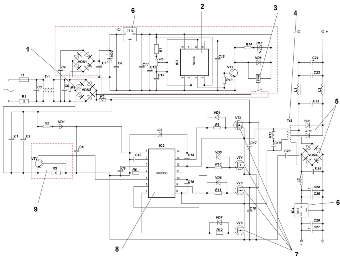
Рис. 1. Вдосконалена схема силових кіл блока живлення лабораторного стенда
