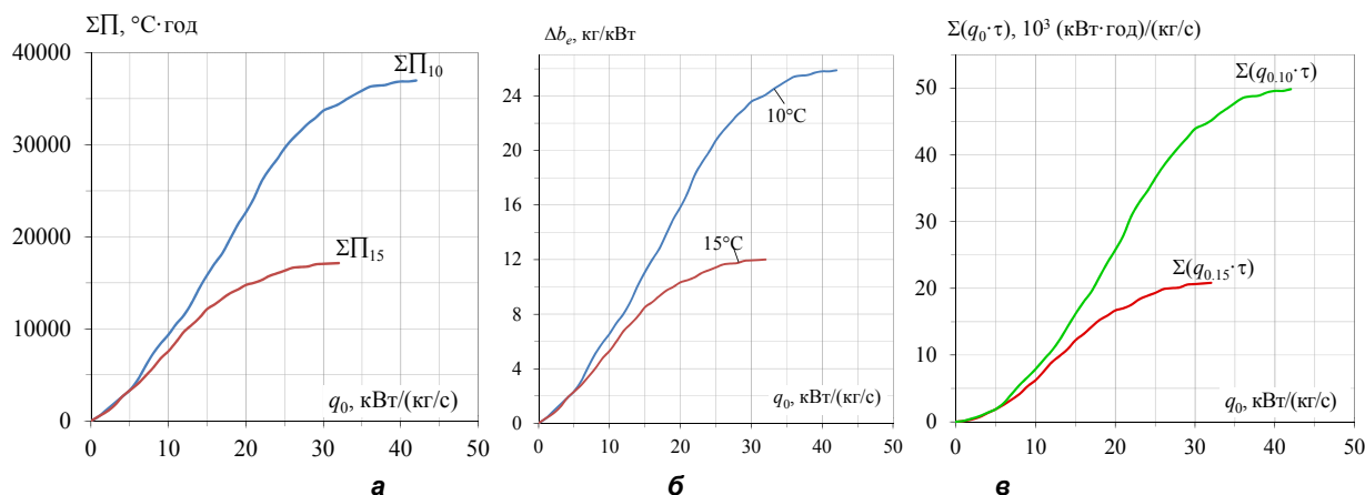
Рис. 1. Значення річного термочасового потенціалу охолодження повітря \Sigma \Pi (а), зменшення питомої витрати палива \Sigma \Delta b_e за рік, віднесеної до 1 кВт потужності ГТУ (б), та річного питомого виробництва холоду \Sigma(q_0 \cdot t) , віднесеного до одиниці витрати повітря G_n = 1 кг/с (в), в залежності від проектної питомої холодопродуктивності У КП q_0 (при G_n = 1 кг/с) при температурах охолодженого повітря t_{н2} = 10 і 15 °C за 2017 р.
