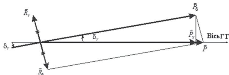
Рис. 1. Схема сил, створених рушієм при перекидці стерна
