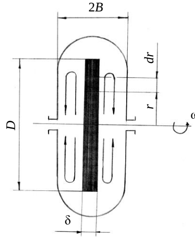
Рис. 2. До розрахунку потужності тертя обертального диска
