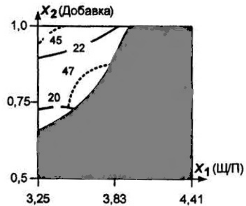
Рис. 3 – Підбір оптимального складу бетону
