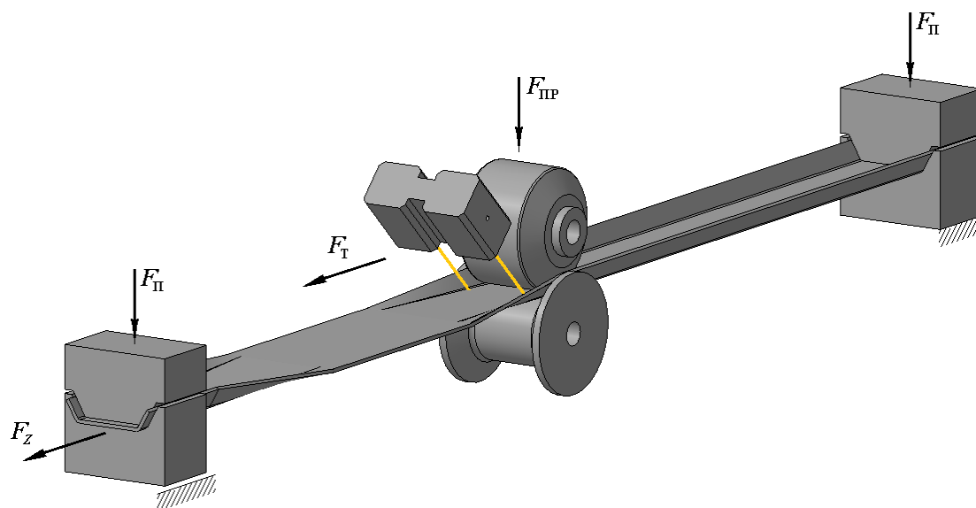
Рисунок 1 – Технологічний процес виготовлення профілю з локальним нагрівом ділянок заготовки лазерним випромінюванням
