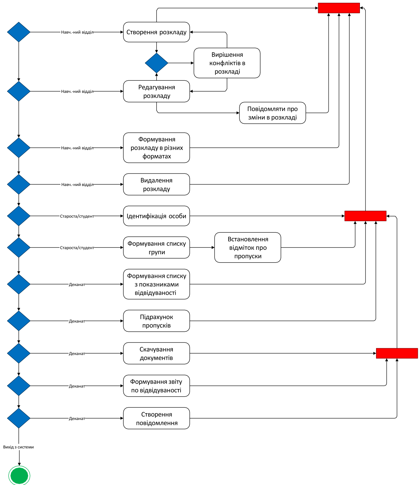
Рисунок 2.7 - Діаграма діяльності
