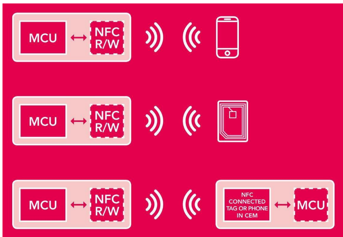
Рисунок 1.4 – Схема режиму читання/запису NFC-пристрою
