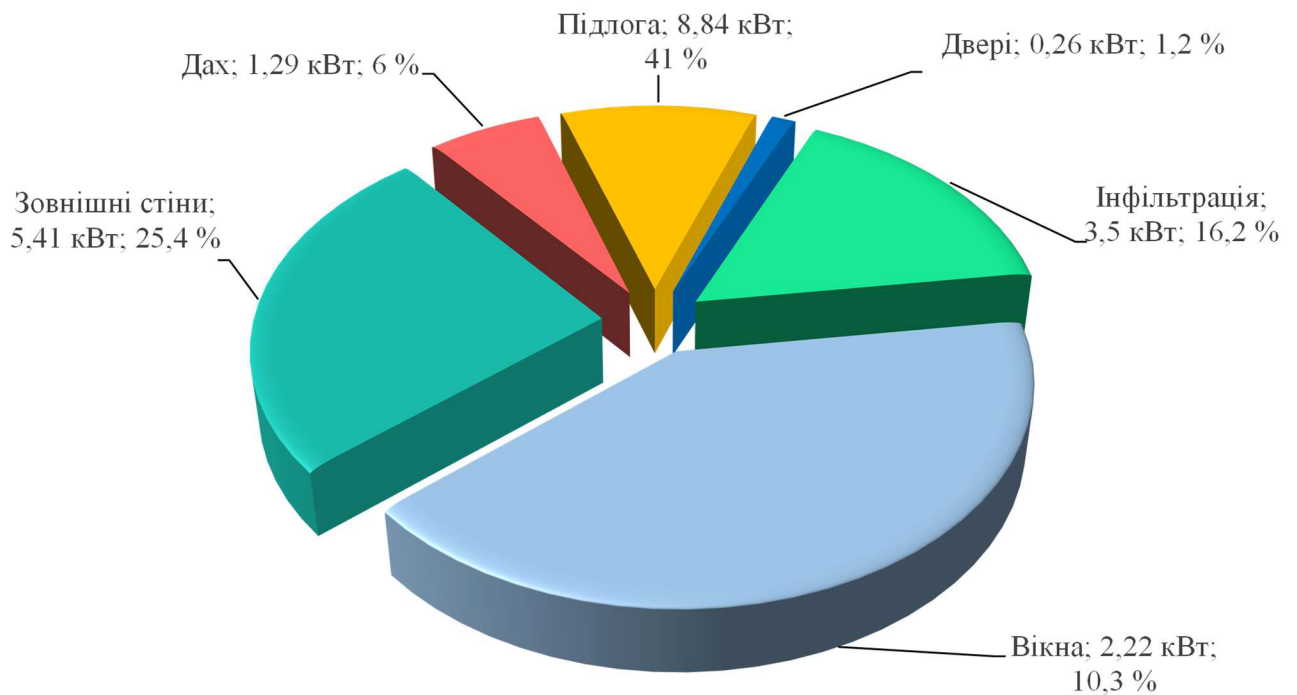
Рис. 3.16. Розподіл існуючих теплових втрат в корпусі будівлі
