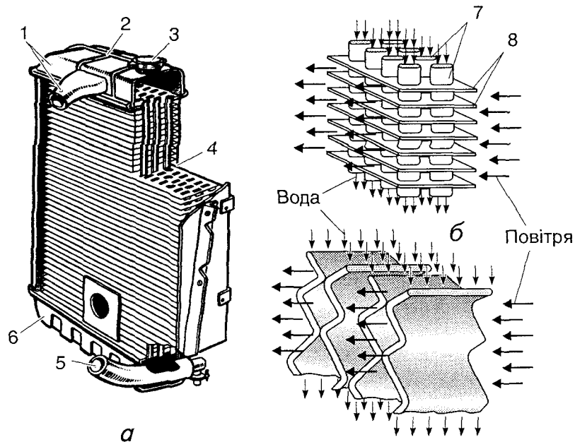
Рисунок 3.2 Радіатор.
