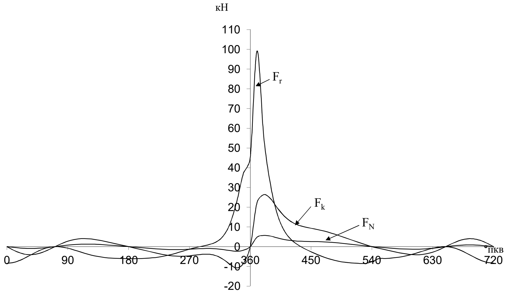
Рисунок 2.2 Сили: радіальна ( F_r ), дотична ( F_k ), нормальна( F_N )
