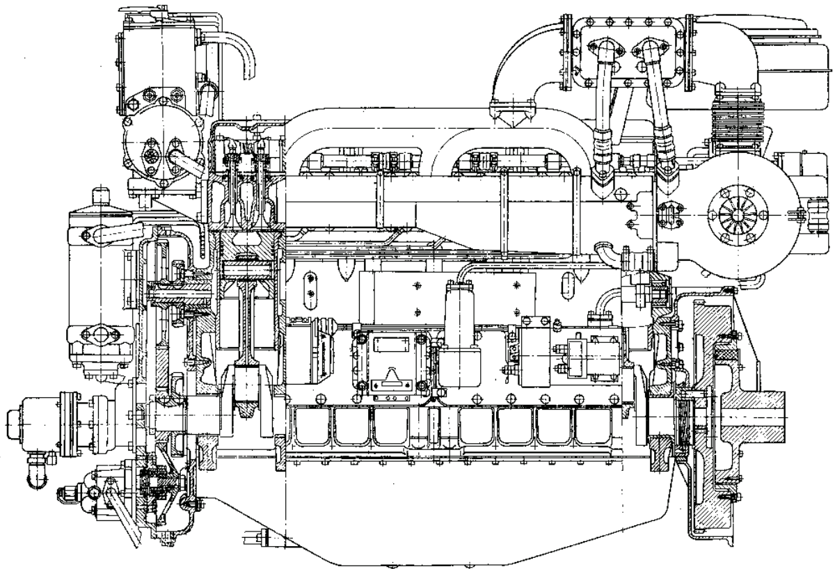
Рисунок 1.3 Повздовжній переріз двигуна 6ГЧН 12/14.
