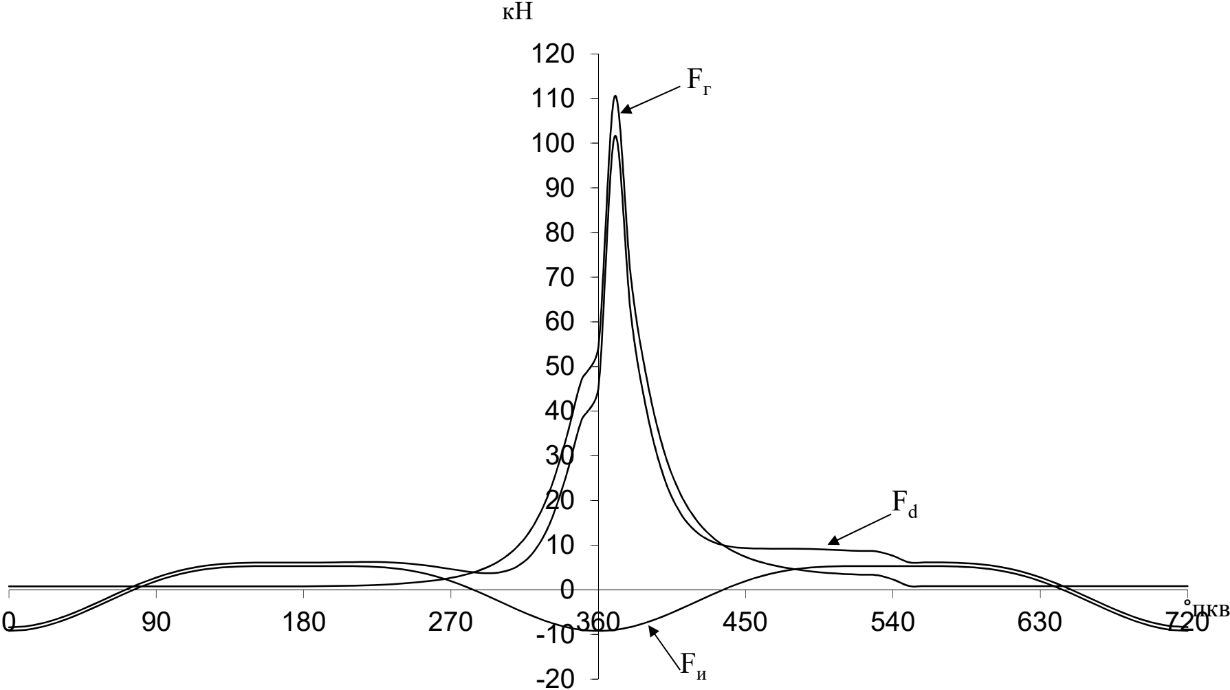
Рисунок 2.1 Сили: газів ( F_g ), інерції ( F_i ), дійсна ( F_d )
