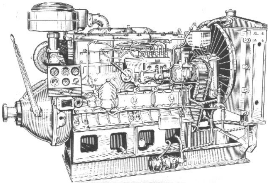
Рисунок 1.1 Загальний вигляд двигуна 6ГЧН 12/14.
