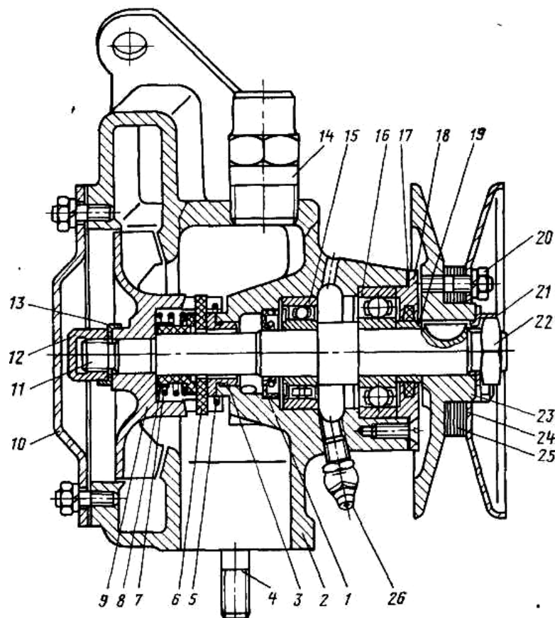
Рисунок 3.4 Водяний насос:
