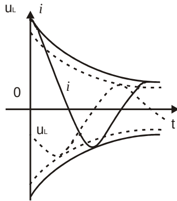
Рис. 3.24. Характер зміни перехідних струму (в контурі) і напруги (на котушці індуктивності)
