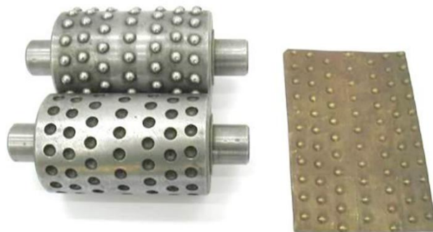
Рисунок 2 – Ролики для профілювання та зразок виготовленої деталі з рельєфом сферичної форми
