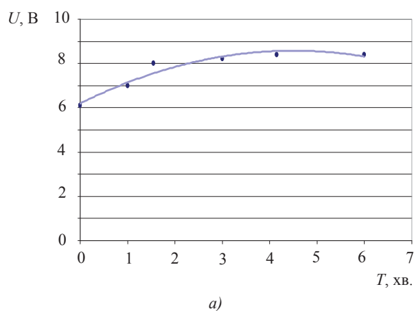
Рис. 2. Динаміка зміни напруги за інтервалу переполюсовки 6 хв. і розміру електродів 25×180 мм:
