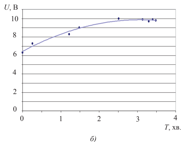
Рис. 2. Динаміка зміни напруги за інтервалу переполюсовки 6 хв. і розміру електродів 25×180 мм:
