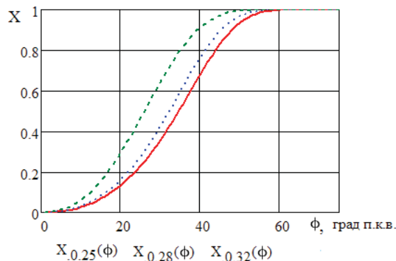
Рис. 3. Частка вигорілого палива в залежності від величини добавки синтез-газу до бензину
