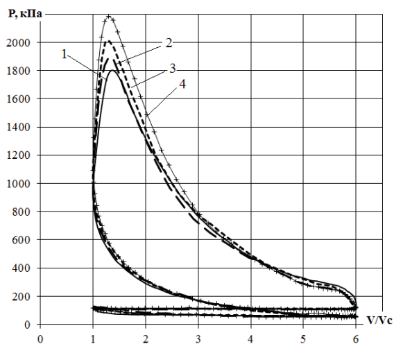
Рис. 1. Індикаторна діаграма двигуна 2С 7,2/6 при різних добавках синтез-газу до бензину: 1 – бензин; 2, 3, 4 – добавка синтез-газу 28%, 32% і 64% відповідно
