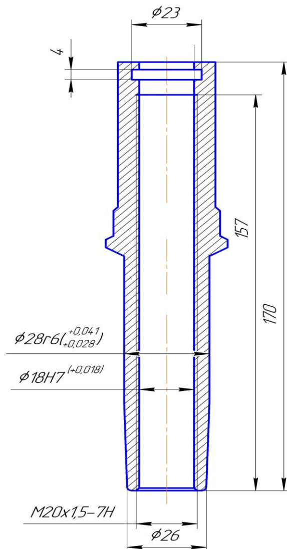
Рисунок 3.7 Втулка направляюча впускного клапана
