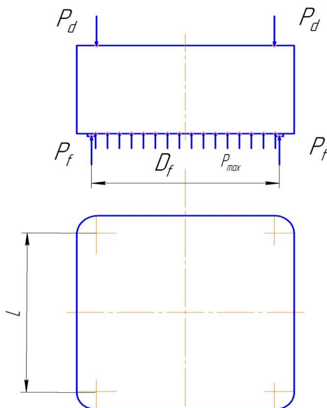
Рисунок 3.8 Розрахункова схема кришки робочого циліндру
