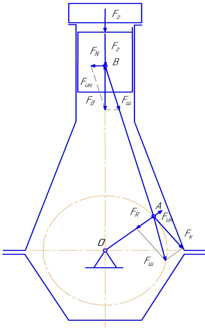
Рисунок 2.1 Схема КШМ та сили, що діють в ньому
