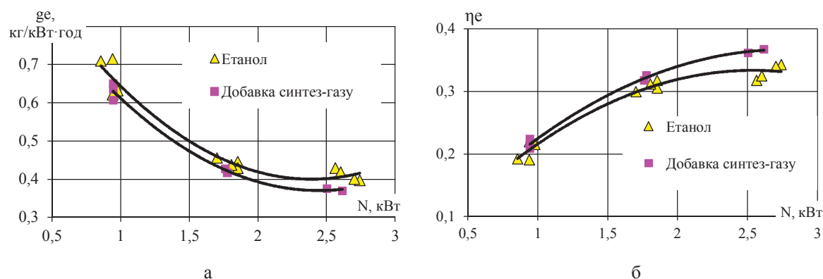
Рис. 3. Основні параметри двигуна при роботі по навантажувальній характеристиці на чистому етанолі і з добавкою синтез-газу:
