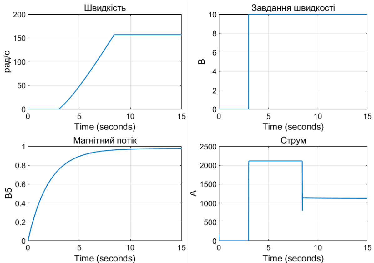
Рис. 2. Перехідні характеристики
