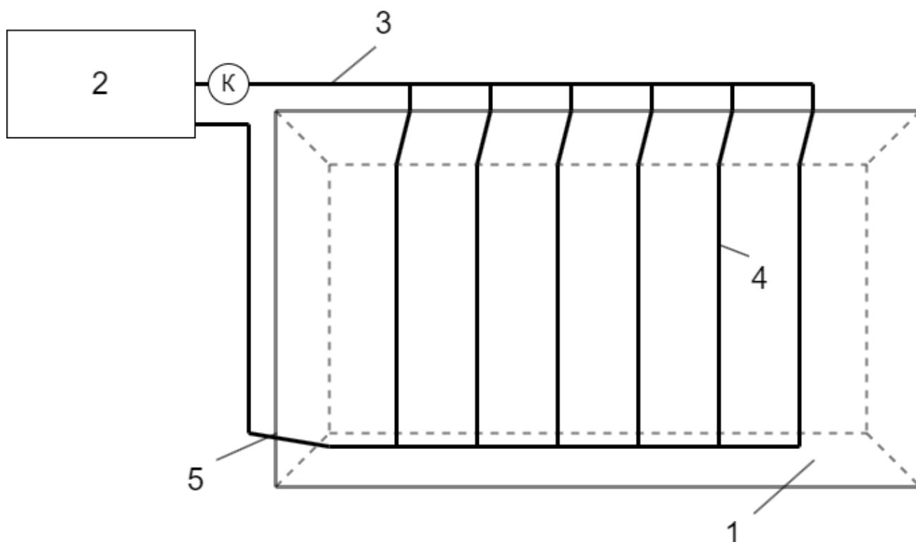
Рис. 5.6 – Схема дренажу ділянки (1 – ділянка розміщення ЗНІ; 2 – джерело водопостачання; 3 – трубопровід; 4 – система поливу)
