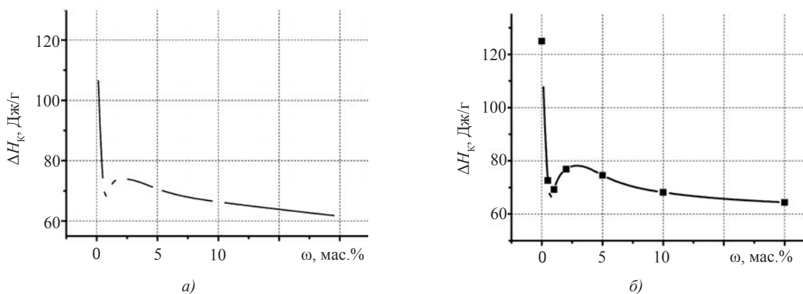
Рис. 3. Залежність ентальпії кристалізації від відсоткового вмісту вуглецевих нанотрубок у поліпропілені при швидкості охолодження: а) \bar{v}_t = 1 К/хв ; б) \bar{v}_t = 5 К/хв.
