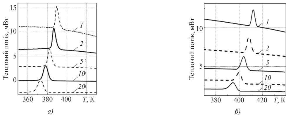
Рис. 1. Екзотерми кристалізації для ПП-0 (а) і ПП-20 (б) при різних значеннях швидкостей охолодження: 1 — \bar{v}_t = 1 ; 2 — \bar{v}_t = 2 ; 3 — \bar{v}_t = 5 ; 4 — \bar{v}_t = 10 ; 5 — \bar{v}_t = 20 К/хв.
