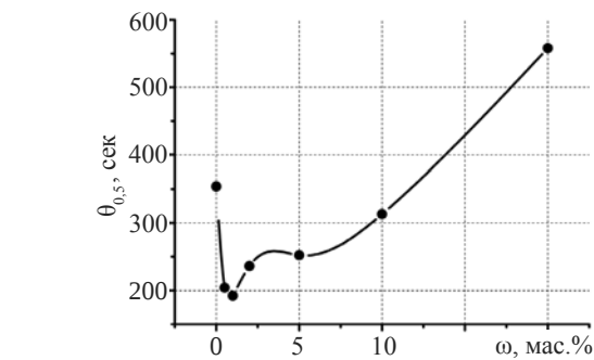
Рис. 4. Залежність періоду напівкристалізації від процентного вмісту вуглецевих нанотрубок в поліпропілені при швидкості охолодження \bar{v}_c = 1 К/хв.
