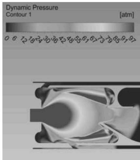
Рис.2. Зображення усіченого конуса факела в епіорах динамічного тиску
