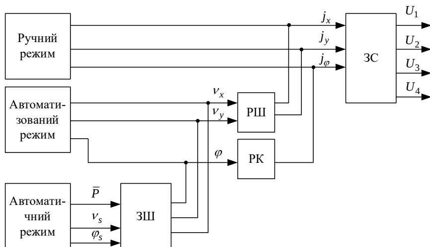
Рисунок 2 – Система керування рухом СБПП
