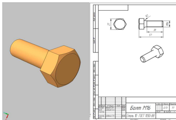
Рисунок 5 – 3D-модель болта і кресленик, виконані в "Компас"
