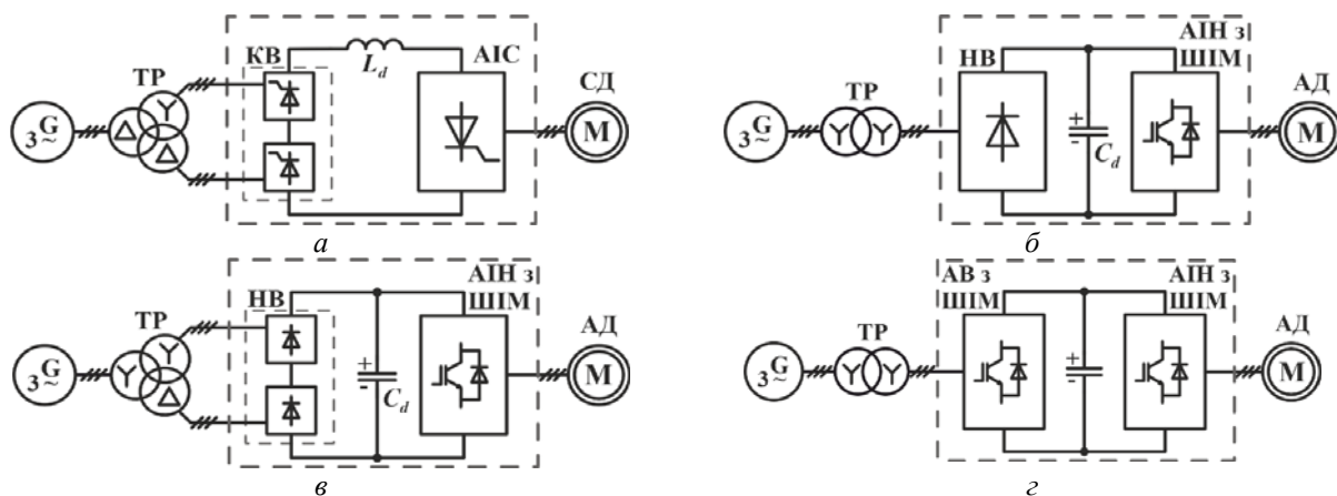
Рис. 1. Основні структури перетворювачів частоти, які використовуються в сучасних суднових НПК за типами вхідних перетворювачів: а – з 12-пульсним KB та ALC ; б – з 6-пульсним HB та АІН з ШІМ ; в – з 12-пульсним HB та АІН з ШІМ ; г – з АВ та АІН з ШІМ
