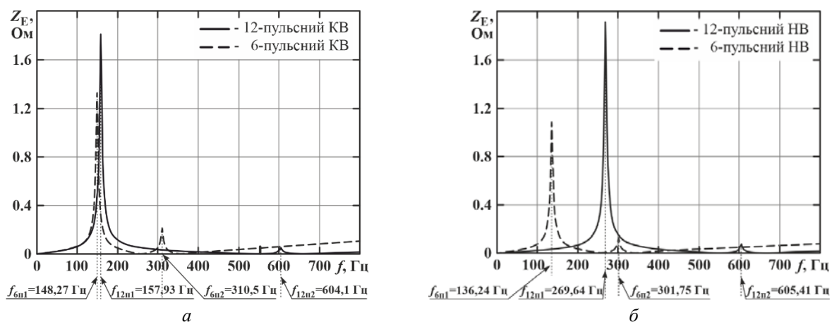
Рис. 7. Частотні характеристики еквівалентного повного опору СЕЕС Z_E(f) з одно- (а) та дволанковими (б) КФКП
