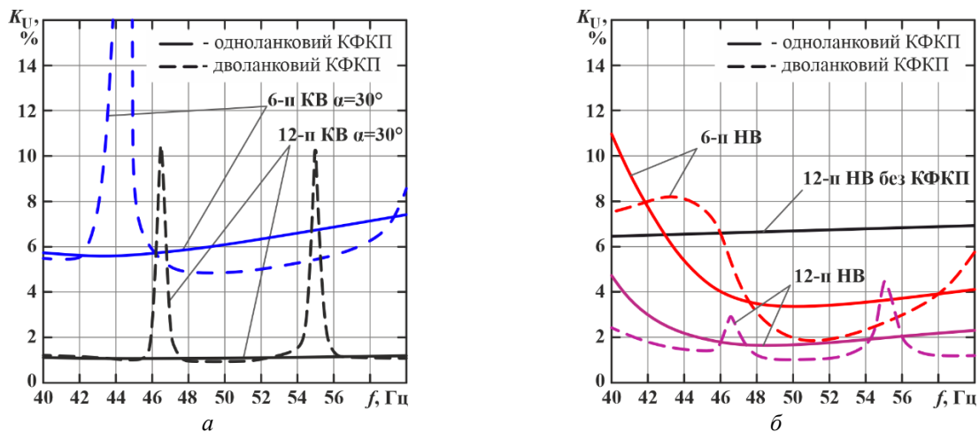
Рис. 6. Залежності K_U від відхилень частоти в діапазоні f = (50 \pm 10) Гц для систем з одно- та дволанковими КФКП: а – при 6- та 12-пульсному вхідному КВ ПЧ; б – при 6- та 12-пульсному вхідному НВ ПЧ
