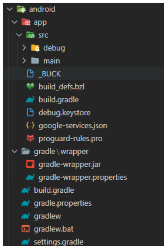
Рисунок 3.3 – Вміст папки android
