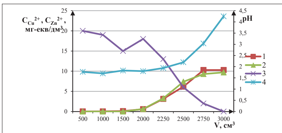
Рис. 3. Залежність вихідної концентрації іонів міді (1), цинку (2), кислотності (3) та pH (4) розчину ( [\text{Cu}^{2+}] = 10,3 мг-екв/дм³; [\text{Zn}^{2+}] = 9,7 мг-екв/дм³; [\text{SO}_4^{2-}] = 20 мг-екв/дм³) при фільтруванні його через катіоніт КУ-2-8 в кислій формі ( V_i = 20 см³) (ПОДС 1 = 1152,16 мг-екв/дм³, ПОДС 2 = 1068,33 мг-екв/дм³)
