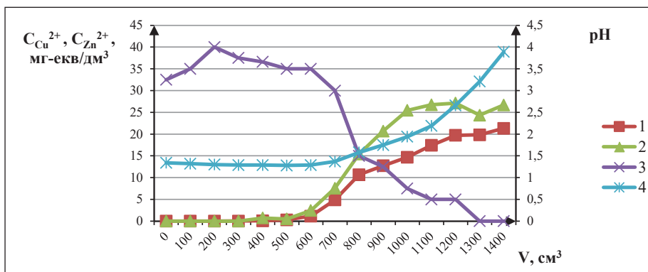
Рис. 2. Залежність вихідної концентрації іонів міді (1), цинку (2), кислотності (3) та pH (4) розчину ( [\text{Cu}^{2+}] = 20 мг-екв/дм³; [\text{Zn}^{2+}] = 27,6 мг-екв/дм³; [\text{SO}_4^{2-}] = 48 мг-екв/дм³) при фільтруванні його через катіоніт КУ-2-8 в кислій формі ( V_i = 20 см³) (ПОДС 1 = 926,42 мг-екв/дм³, ПОДС 2 = 1181,2 мг-екв/дм³)
