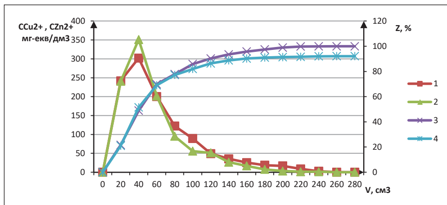
Рис. 4. Залежність вихідних концентрацій іонів міді (1), цинку (2), ступеня десорбції іонів міді (3) та цинку (4) від пропущеного об'єму 10%-го розчину H_2SO_4 через катіоніт КУ-2-8 в Cu^{2+}, Zn^{2+} формі
