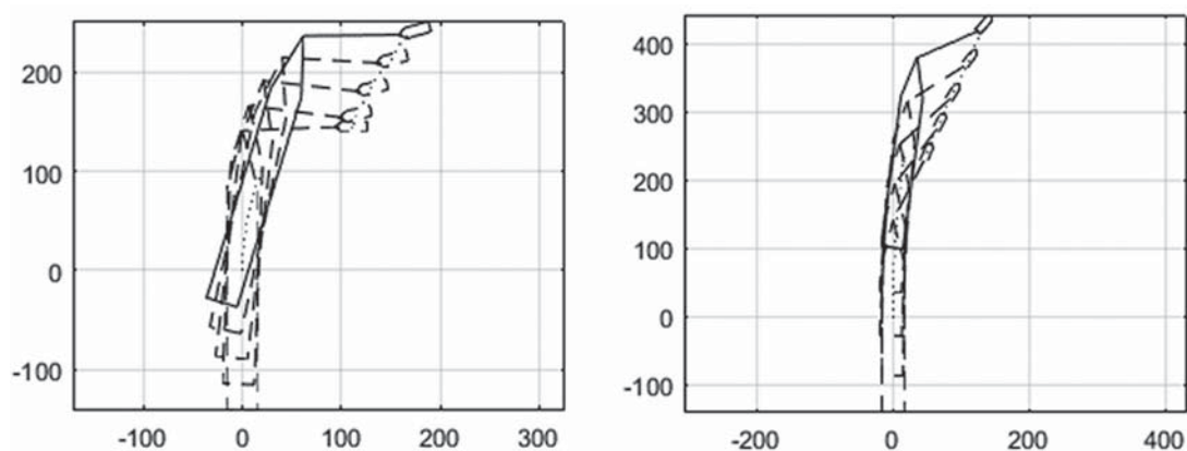
Рис. 3. Моделирование работы системы буксир-судно в различных режимах: слева — «bow-to-bow», скорость — 2 узла; справа — «stern-to-bow», скорость — 4 узла
