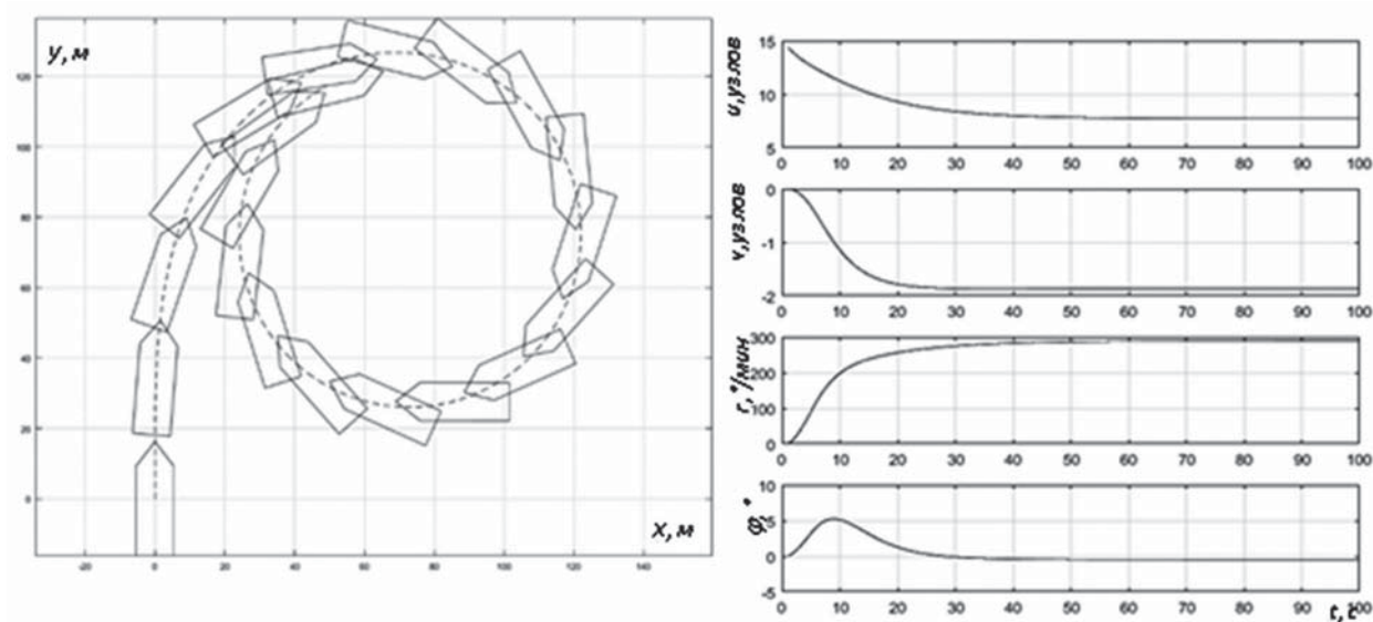
Рис. 2. Циркуляция ASD буксира на правый борт; разворот двигателей 35^\circ
