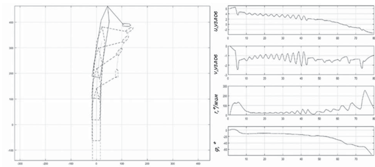
Рис. 4. Моделирование ситуации «гиртинг». Режим «stern-to-bow», скорость — 6 узлов
