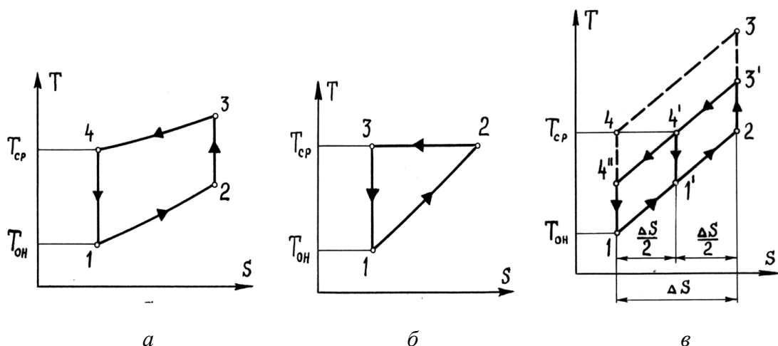
Рисунок 1 - Цикли з неізотермічністю робочого тіла в процесах теплообміну: а – Лоренца; б – трикутний; в – Лоренца 1-2-3-4-1 та ступінчастий 1-1'-2-3'-4'-4''-1
