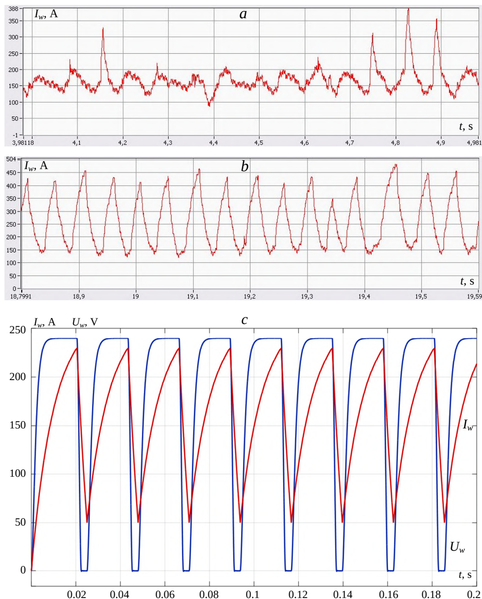
Рис. 4. Сравнительные результаты исследования процесса дуговой сварки и наплавки: a – ток обычного процесса; b – ток процесса с дозированной подачей электродной проволоки; c – моделирование процесса сварки (качественное представление)
