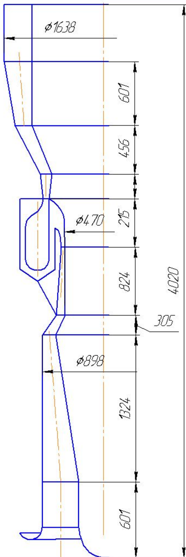
Рис.3.4. Ескіз меридіанного перерізу ГТД
